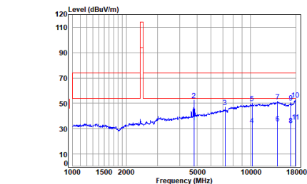
2.4G_SRD_TX_LOW_Horizontal
