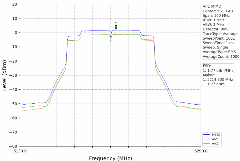
802.11ac(VHT80)_MCH_5210MHz_MIMO_NTNV
