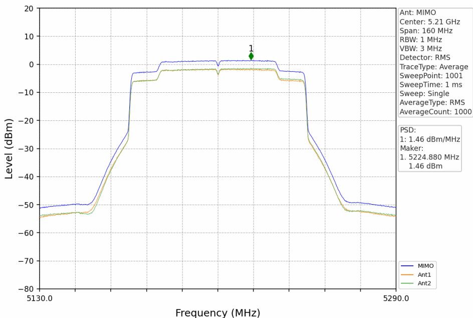
802.11ax(HEW80)_MCH_5210MHz_RU996_Left_MIMO_NTNV
