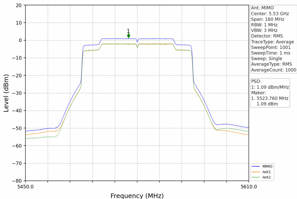
802.11ax(HEW80)_LCH_5530MHz_RU996_Left_MIMO_NTNV
