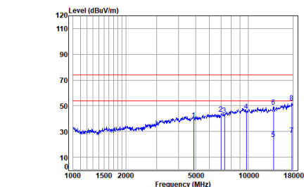
BT_DH5_TX_CH_39_Horizontal
