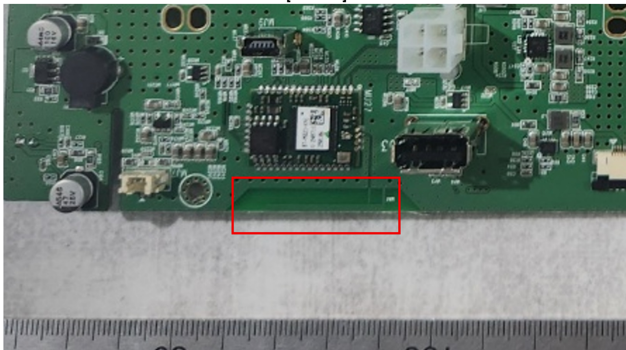
[Antenna]
