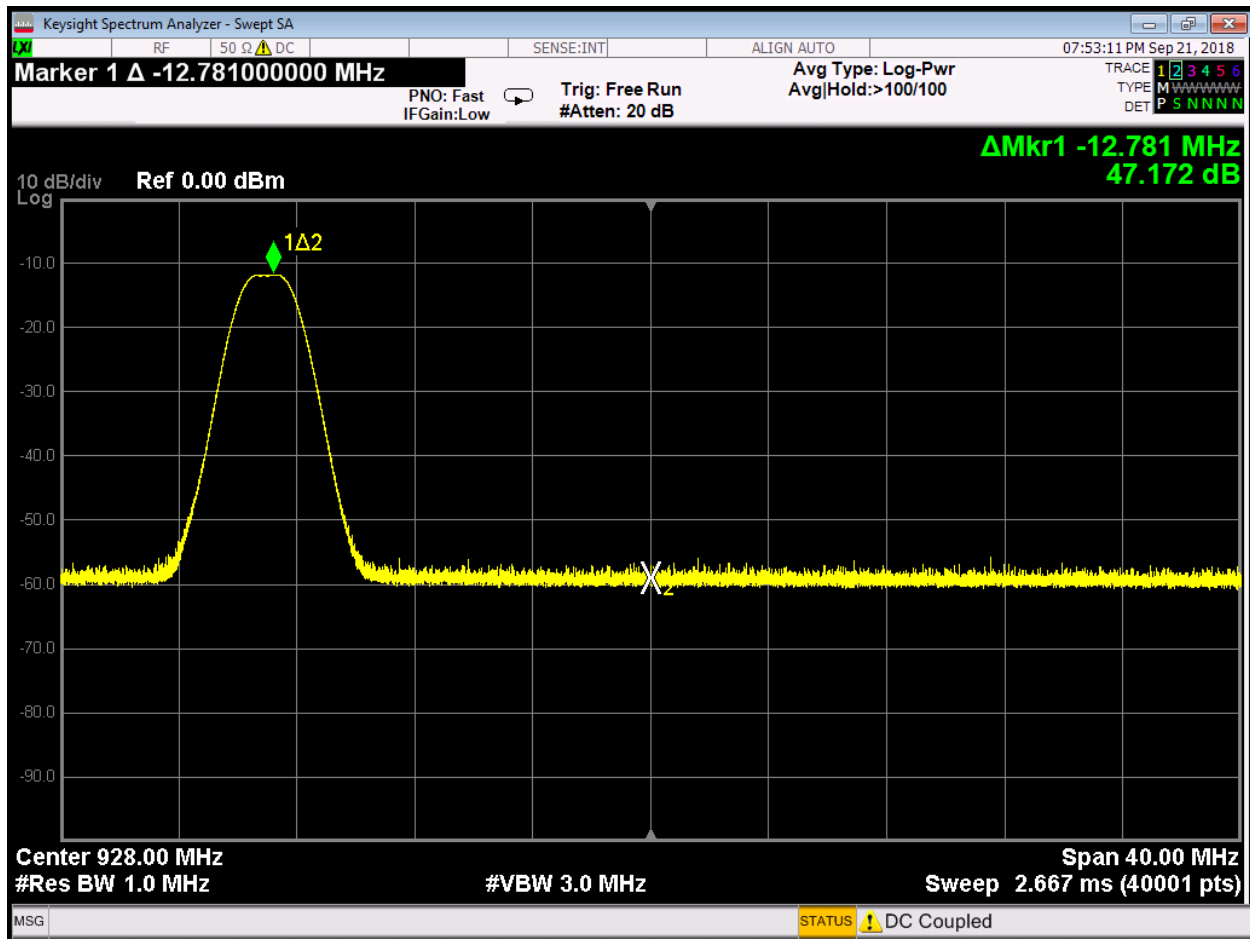
Low Data Rate Upper Band Edge
