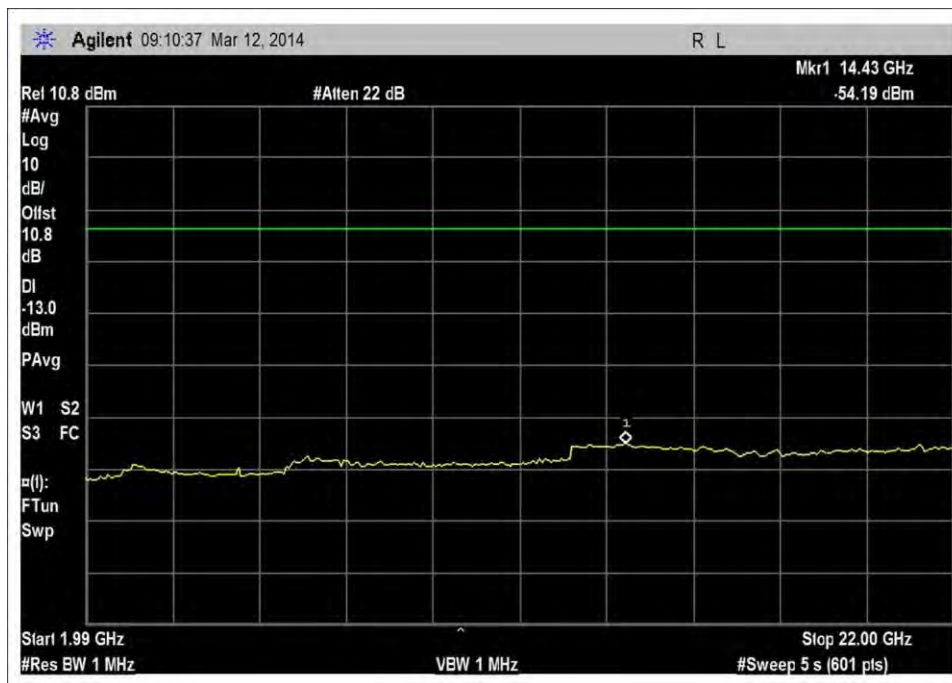
DL_1930-1995MHz_1991-22000MHz
