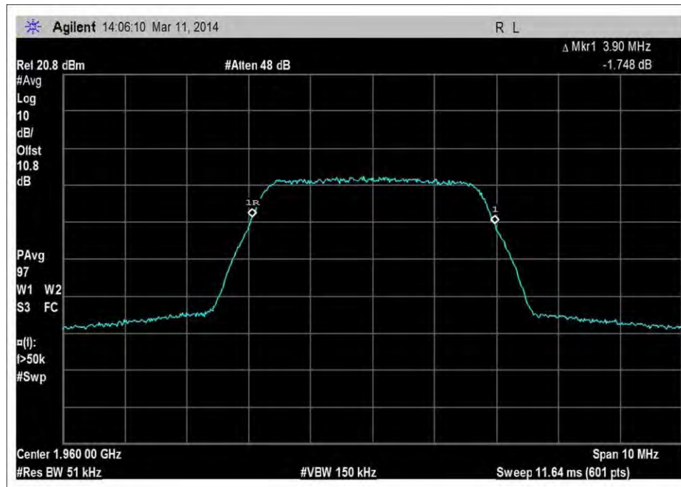
DL_1930-1995MHz_41AWGN_output
