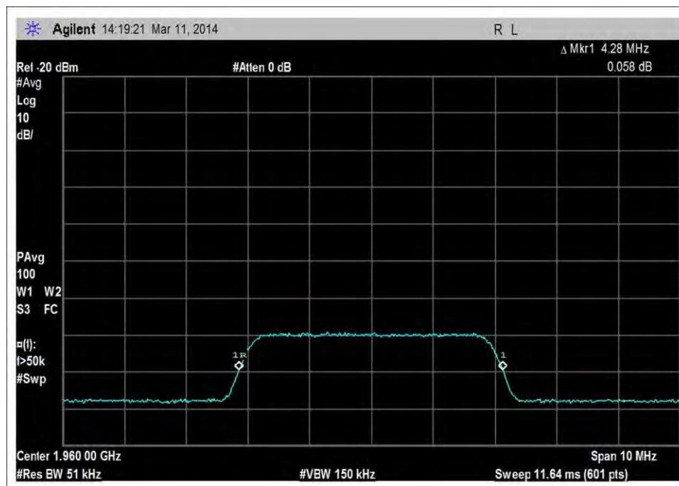
DL_1930-1995MHz_41AWGN_input_-70dBm
