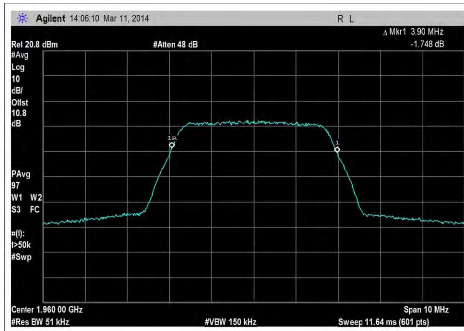
DL_1930-1995MHz_41AWGN_output
