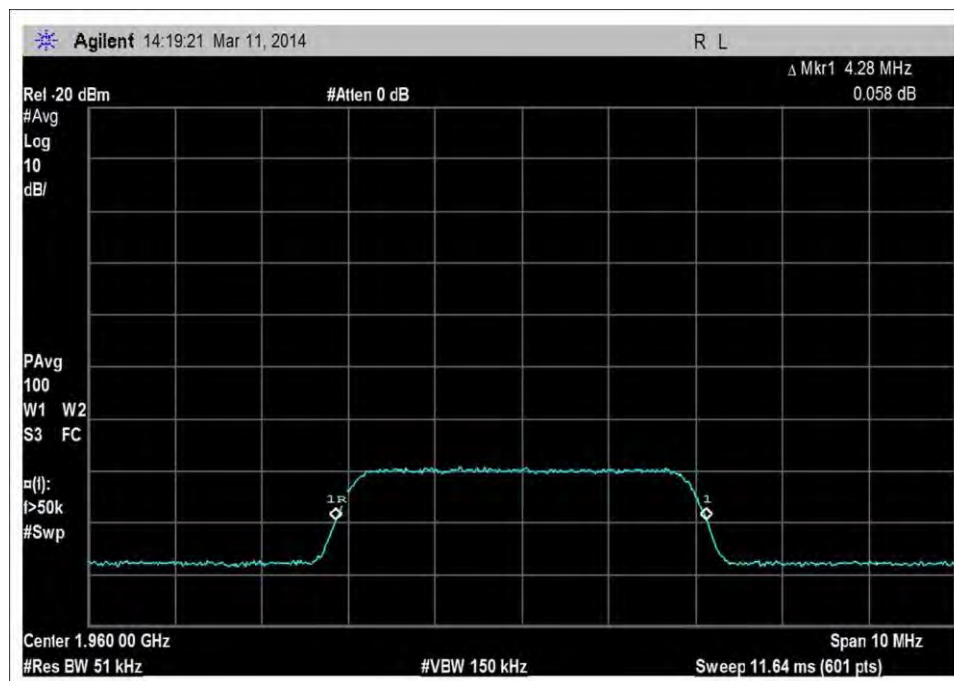
DL_1930-1995MHz_41AWGN_input_-70dBm
