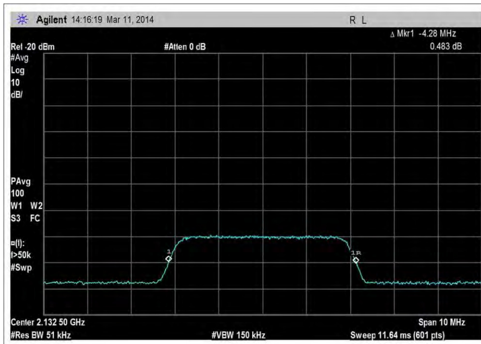
DL_2110-2155MHz_41AWGN_input_-70dBm
