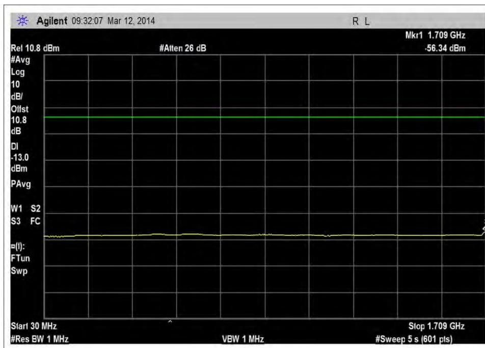
UL_1710-1755MHz_30-1709MHz
