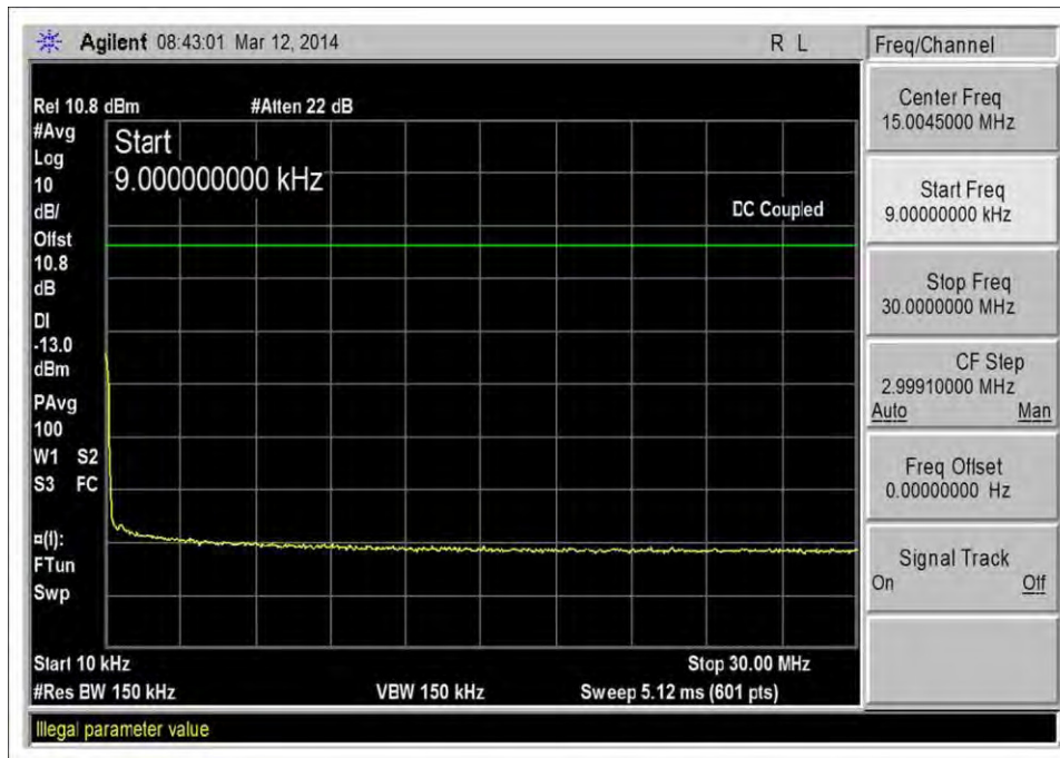
DL_2110-2155MHz_9kHz-30MHz
