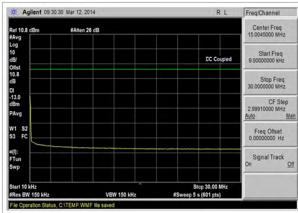
UL_1710-1755MHz_9kHz-30MHz
