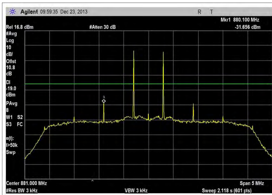
DL_869-894MHz_-75dBm
