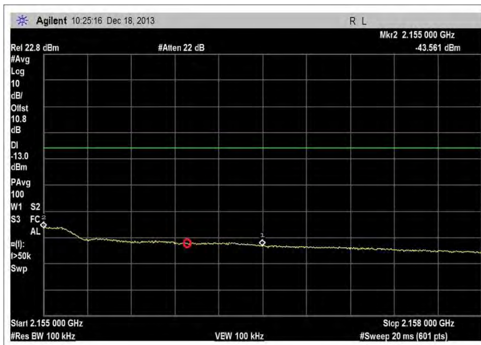
DL_2110-2155MHz_H_-90dBm_rbw100kHz
