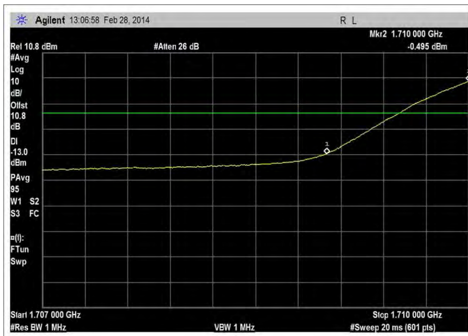
UL_1710-1755MHz_L_RFin_0dBm_rbw=1MHz
