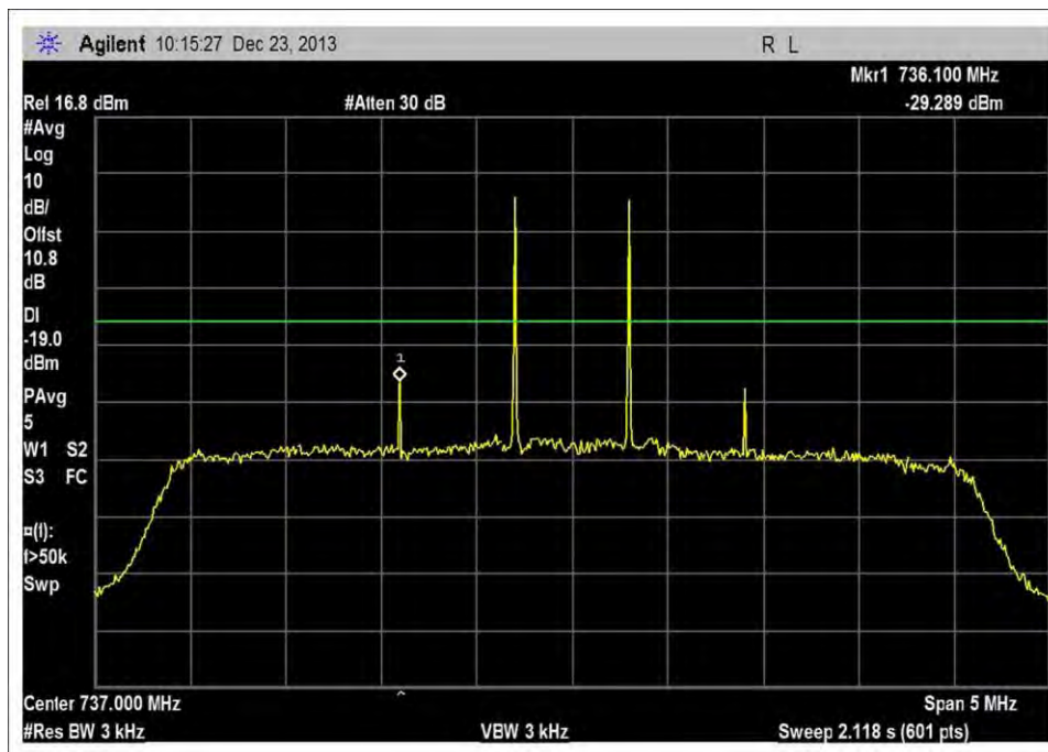
DL_716-746MHz_-85dBm
