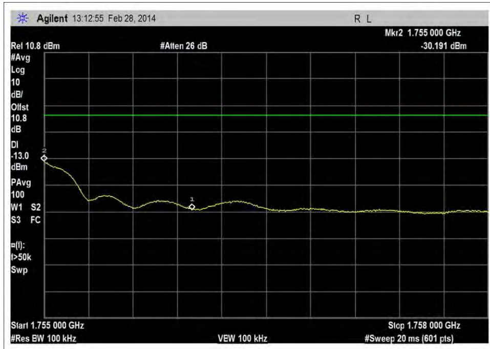
UL_1710-1755MHz_H_RFin -78dBm_rbw=100kHz
