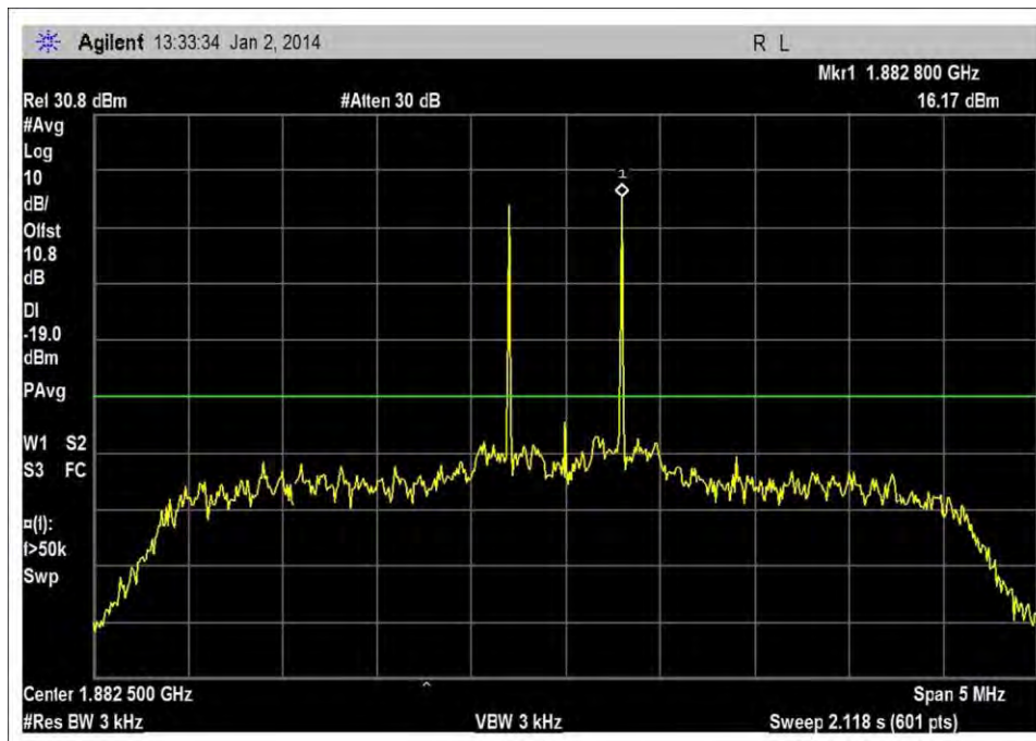
UL_1850-1915MHz_-50dBm
