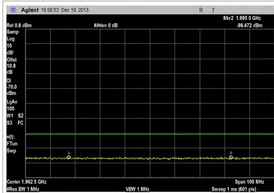
DL_1930-1995MHz_MNC005
