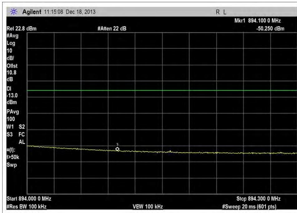
DL_869-894MHz_H_-20dBm
