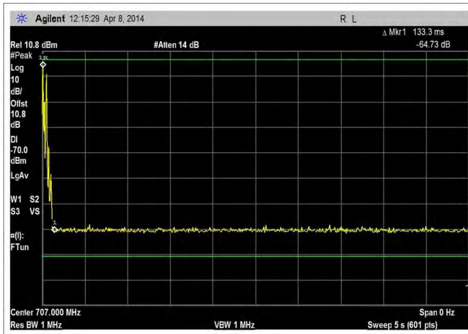
UL_698-716MHz_Single
