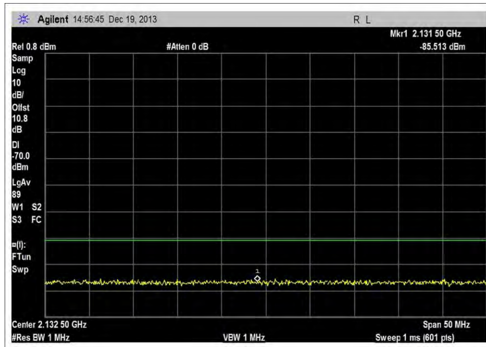
DL_2110-2155MHz_MNC005
