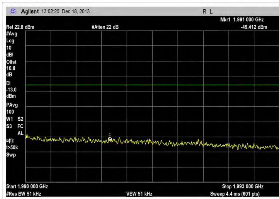
DL_1930-1995MHz_H_-90dBm_rbw51k
