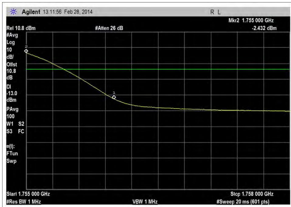
UL_1710-1755MHz_H_RFin -78dBm_rbw=1MHz
