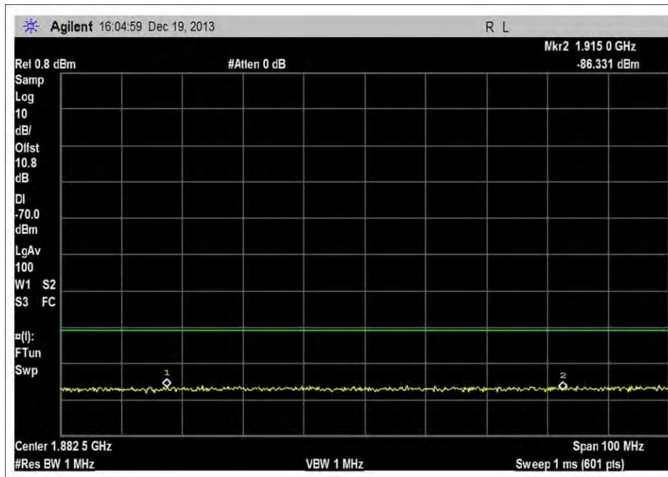
UL_1850-1915MHz_MNC005
