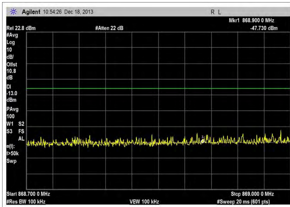
DL_869-894MHz_L_-90dBm
