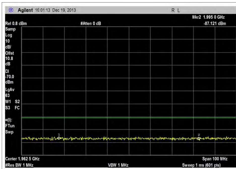
DL_1930-1995MHz_MNC260
