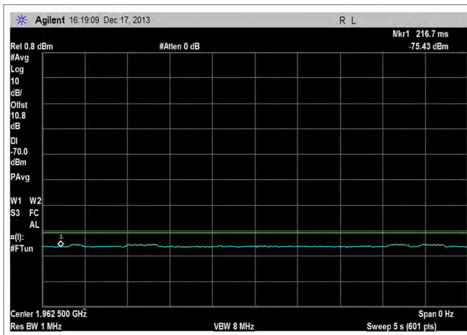
DL_1930-1995MHz_Single-70dBm
