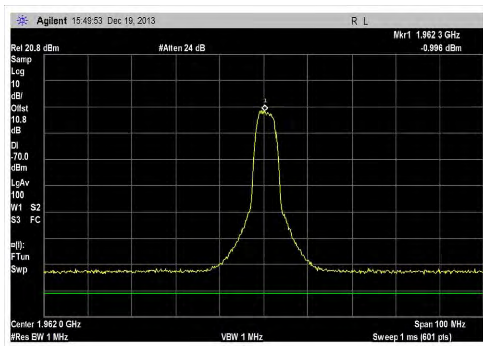
DL_1930-1995MHz_MNC410
