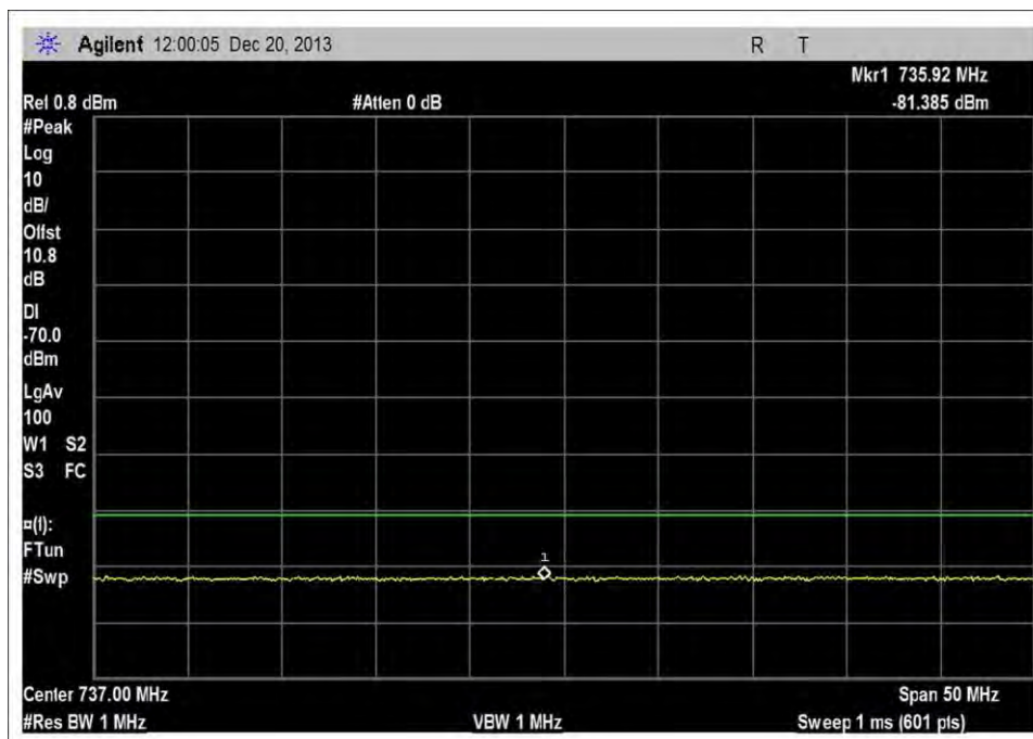
DL_716-746MHz_MNC005
