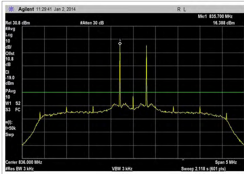
UL_824-849MHz_-60dBm
