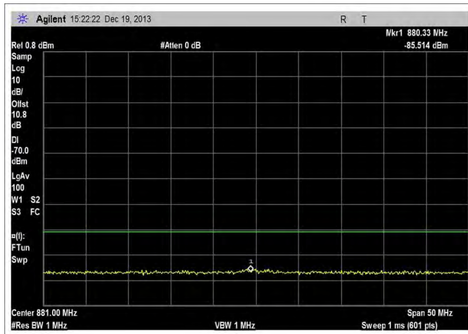
DL_869-894MHz_MNC005
