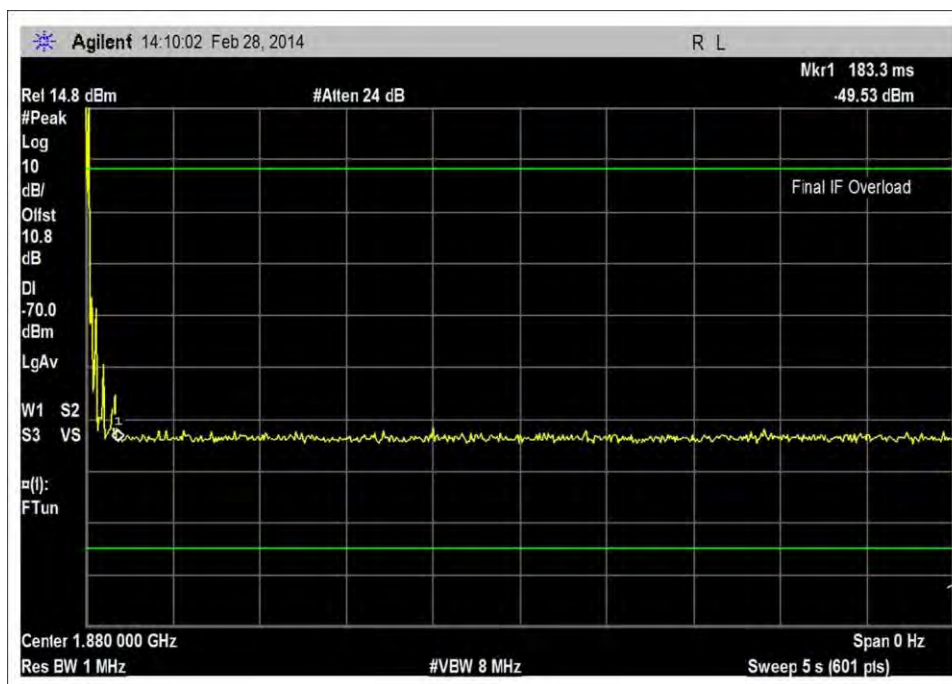
UL_1850-1915MHz_Single
