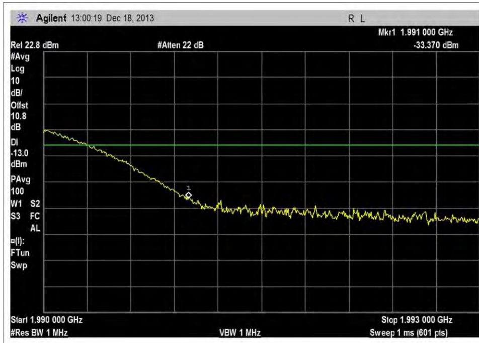
DL_1930-1995MHz_H_-90dBm
