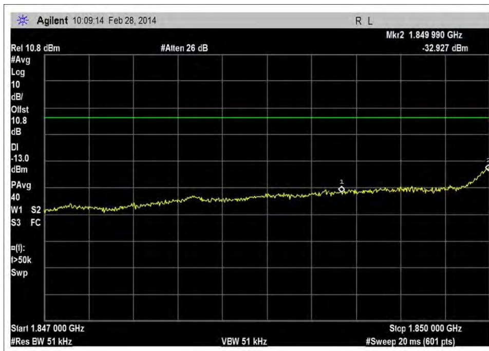
UL_1850-1915MHz_L_RFin 0dBm_rbw=51kHz
