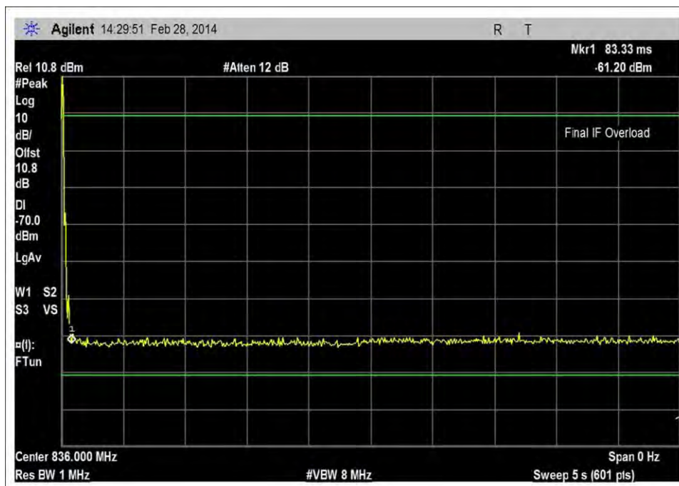
UL_824-849MHz_Single
