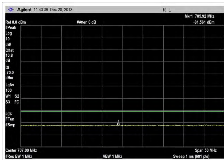
UL_698-716MHz_MNC260
