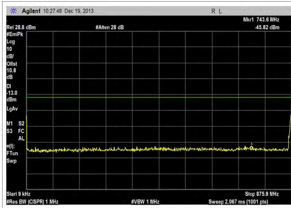
DL_869-894MHz_M_5WCDMA_1
