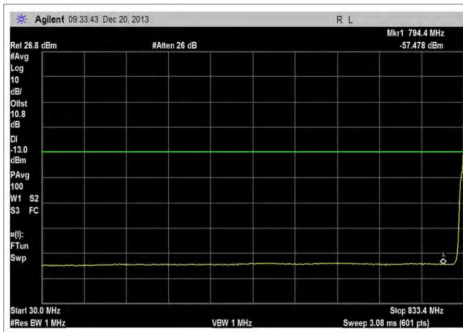
UL_824-849MHz_M_5MWCDMATM1_2
