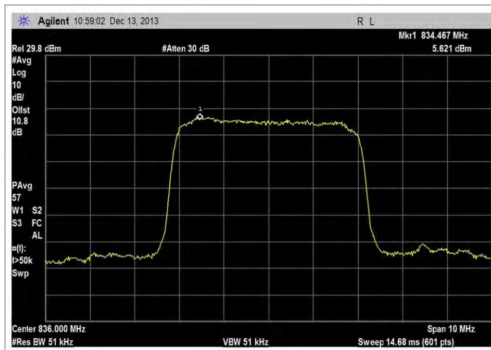
UL_824-849MHz_Output
