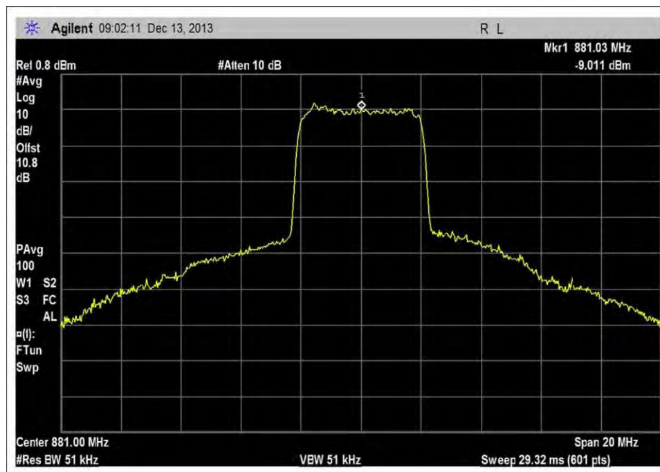
DL_869-894MHz_Output
