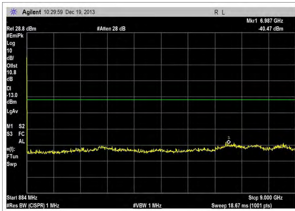
DL_869-894MHz_M_5WCDMA_2
