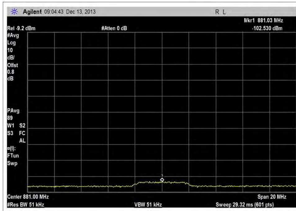
DL_869-894MHz_Input
