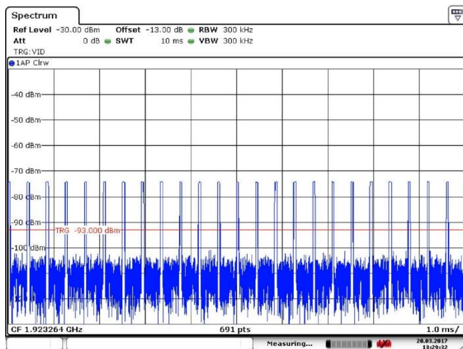
50 µs Pulses
