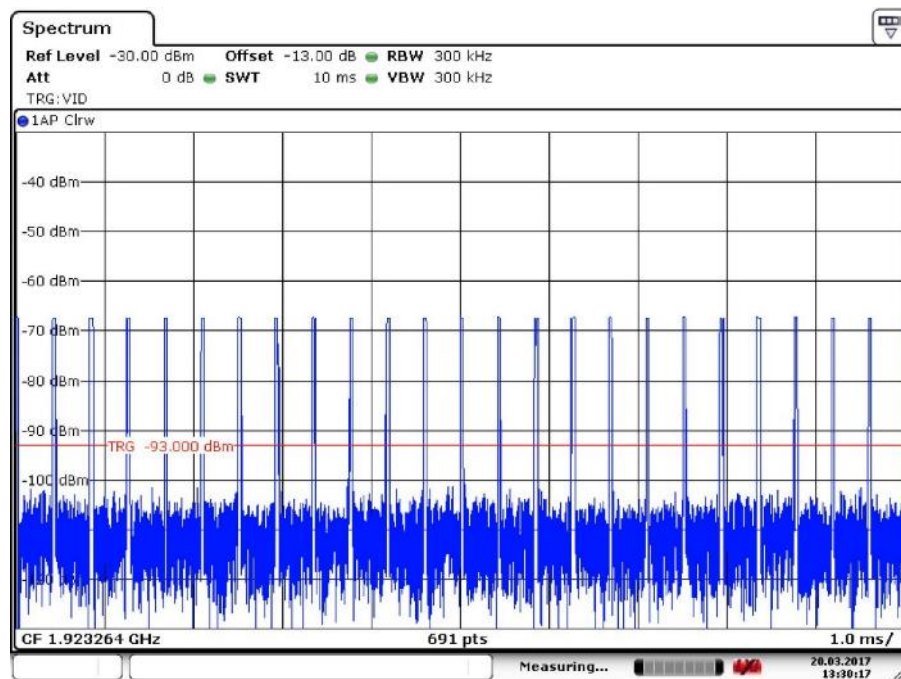
35 µs Pulses
