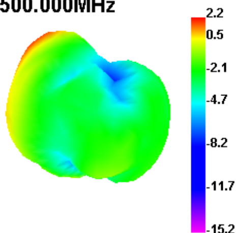
2500.000MHz E1
