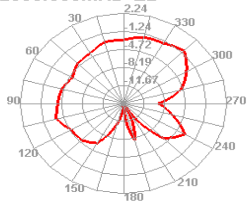
2500.000MHz E2
