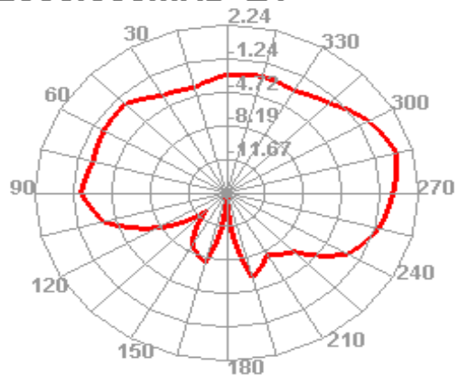
2500.000MHz E1
