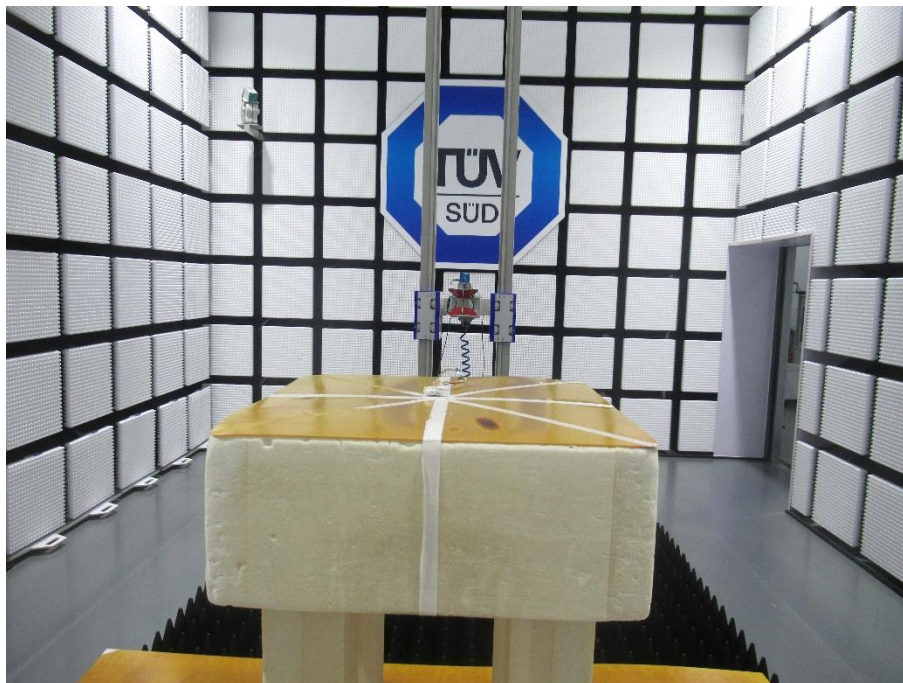
1GHz-18GHz RSE Setup
