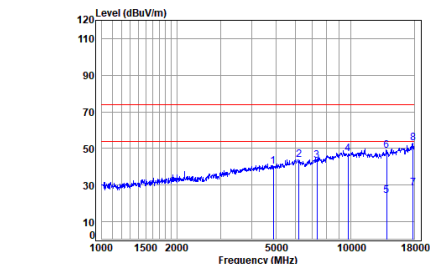
BT_DH5_TX_CH_39_Horizontal
