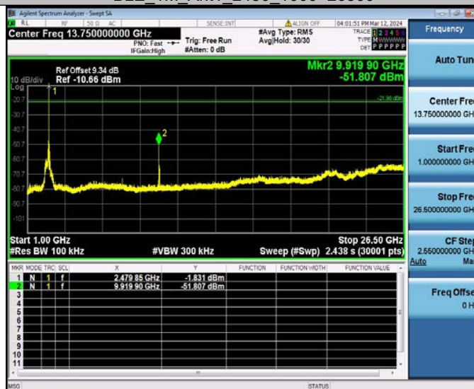
BLE_1M_Ant1_2480_1000~26500
