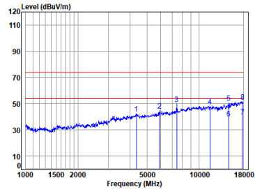
2.4G SRD_TX_CH_78_Vertical
