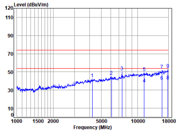
2.4G SRD_TX_CH_78_Horizontal
