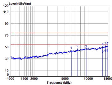
2.4G SRD_TX_CH_39_Horizontal
