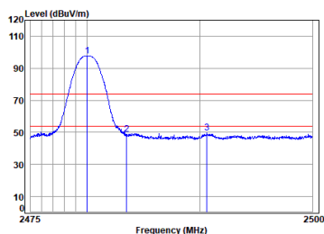
2.4G SRD_TX_CH_78_Horizontal
