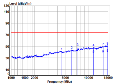
2.4G SRD_TX_CH_39_Vertical
