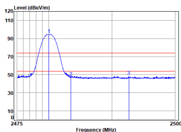
2.4G SRD_TX_CH_78_Vertical
