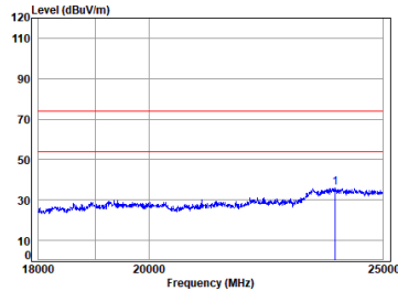
2.4G SRD_TX_CH_78_Horizontal
