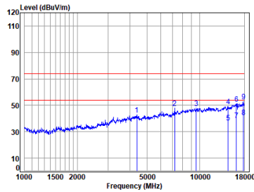
2.4G SRD_TX_CH_00_Horizontal
