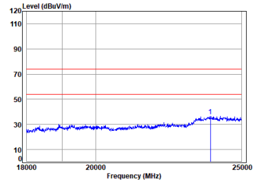
2.4G SRD_TX_CH_78_Vertical
