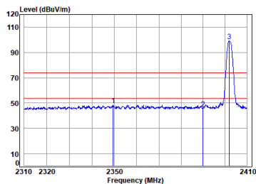
2.4G SRD_TX_CH_00_Horizontal
