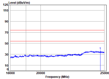
2.4G SRD_TX_CH_00_Horizontal
