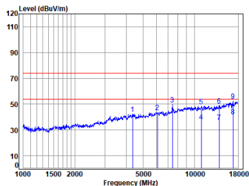
BLE_2M_TX_CH_39_Horizontal
