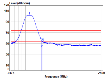
BLE_2M_TX_CH_39_Vertical
