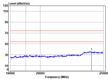
BLE_2M_TX_CH_39_Horizontal
