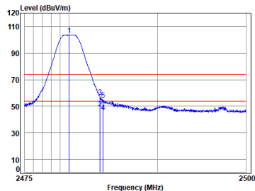
BLE_2M_TX_CH_39_Horizontal
