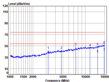
BLE_2M_TX_CH_39_Vertical
