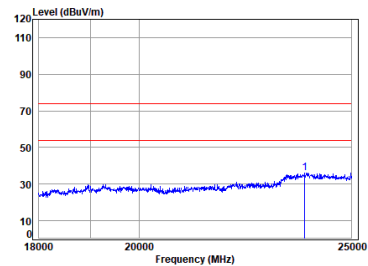
BLE_2M_TX_CH_39_Vertical
