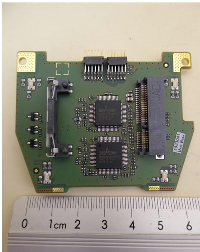
Data PCB Bottom
