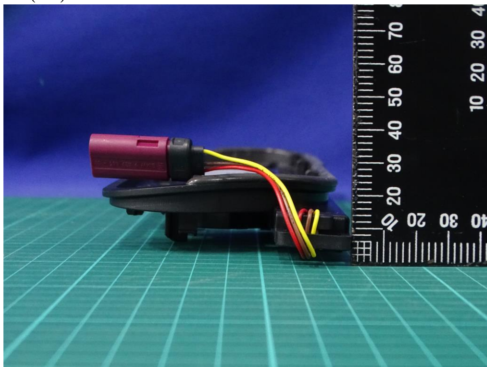
(12) EUT Photo (G70)
