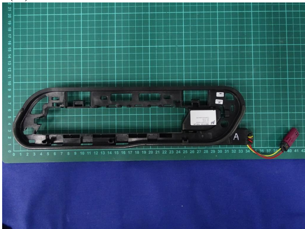
(1) EUT Photo (I20)
