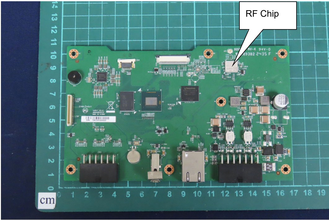
(14) EUT Photo
