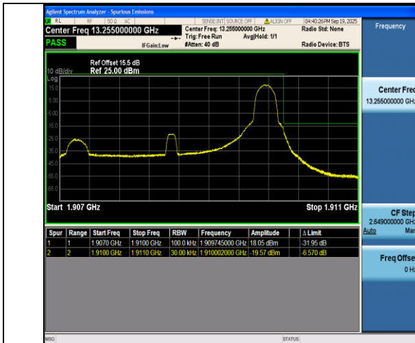
Band2-3MHz-QPSK-19185-1RB#14-PASS
