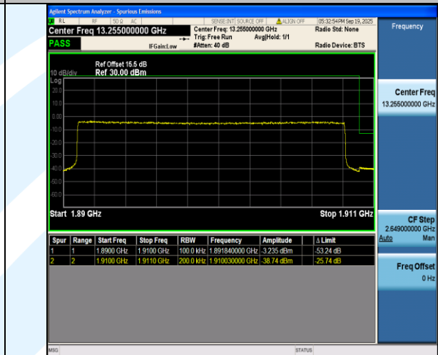
Band2-20MHz-QPSK-19100-100RB#0-PASS
