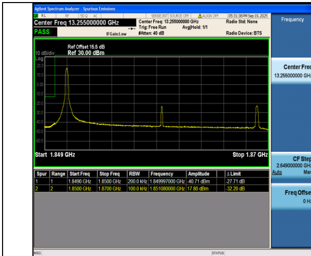
Band2-20MHz-QPSK-18700-1RB#0-PASS
