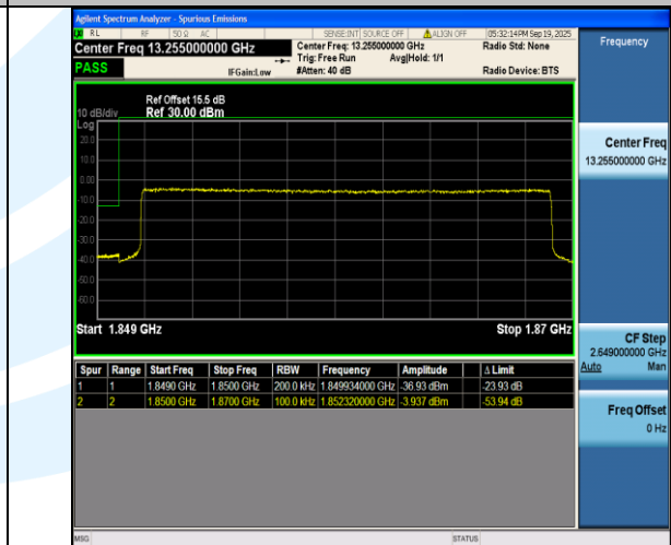
Band2-20MHz-16QAM-18700-100RB#0-PASS
