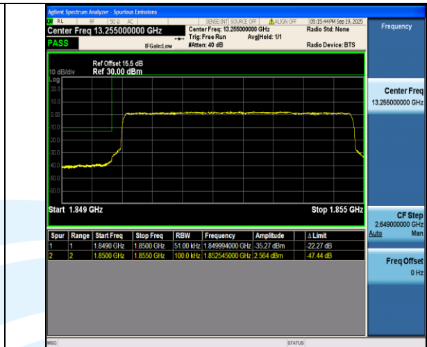
Band2-5MHz-QPSK-18625-25RB#0-PASS
