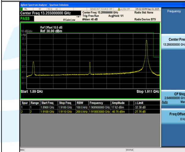
Band2-20MHz-QPSK-19100-1RB#99-PASS
