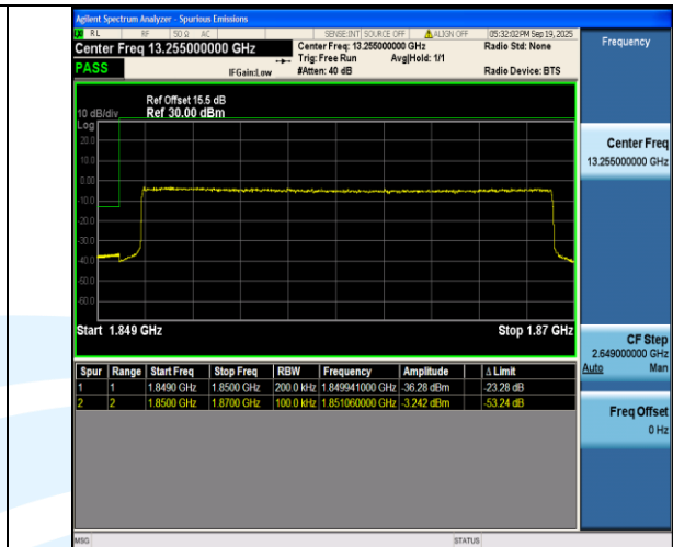
Band2-20MHz-QPSK-18700-100RB#0-PASS
