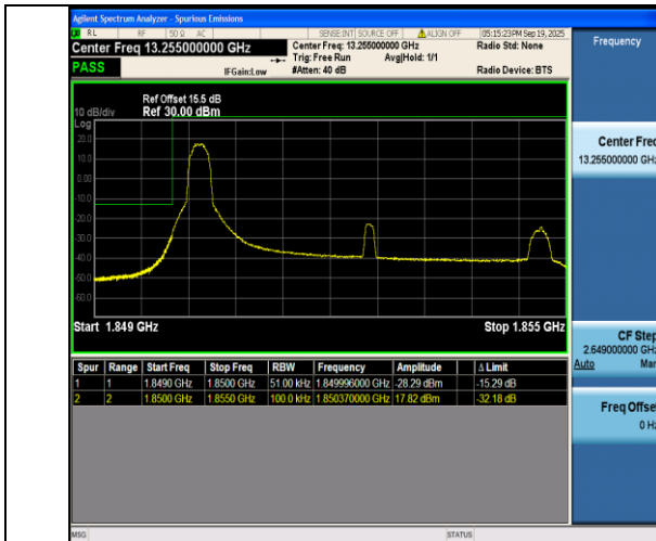
Band2-5MHz-QPSK-18625-1RB#0-PASS
