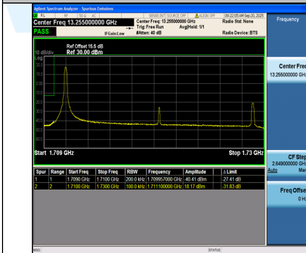
Band66-20MHz-QPSK-132072-1RB#0-PASS
