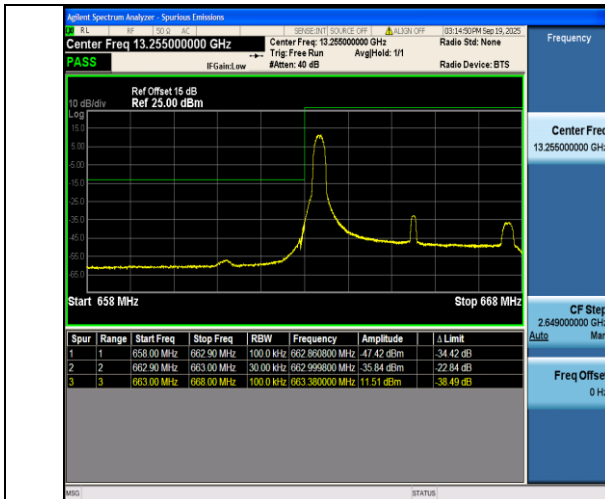
Band71-5MHz-QPSK-133147-1RB#0-PASS
