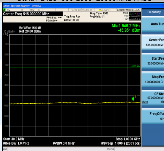
Band4-1513--999-30~1000MHz-PASS
