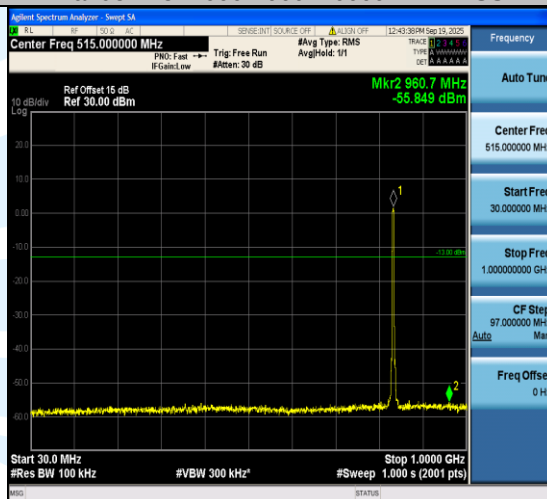
Band5-4182--999-30~1000MHz-PASS
