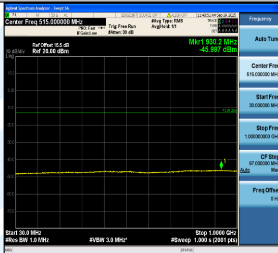
Band2-9538--999-30~1000MHz-PASS
