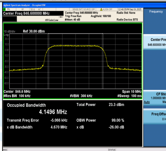
Band5-4233--999-PASS
