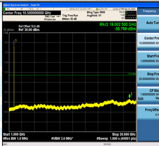
Band4-1513--999-1000~20000MHz-PASS
