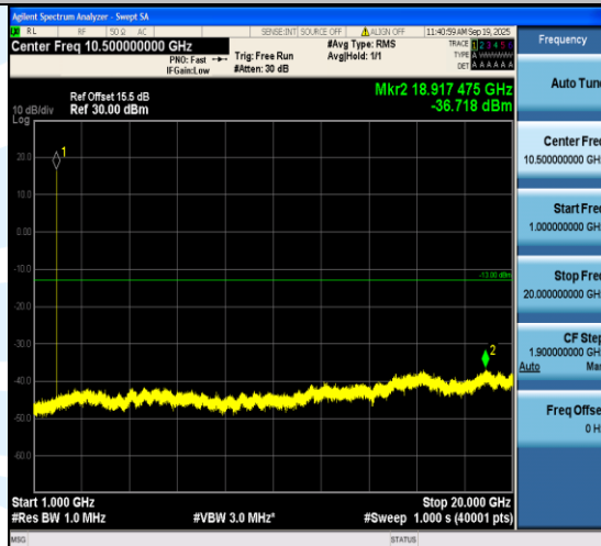
Band2-9538--999-1000~20000MHz-PASS
