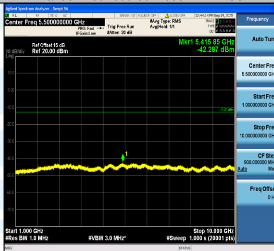
Band5-4233--999-1000~10000MHz-PASS
