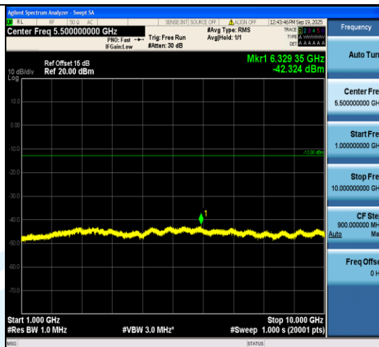
Band5-4182--999-1000~10000MHz-PASS
