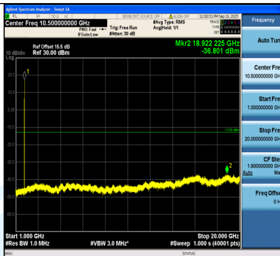
Band4-1413--999-1000~20000MHz-PASS
