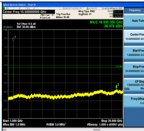
Band2-9400--999-1000~20000MHz-PASS
