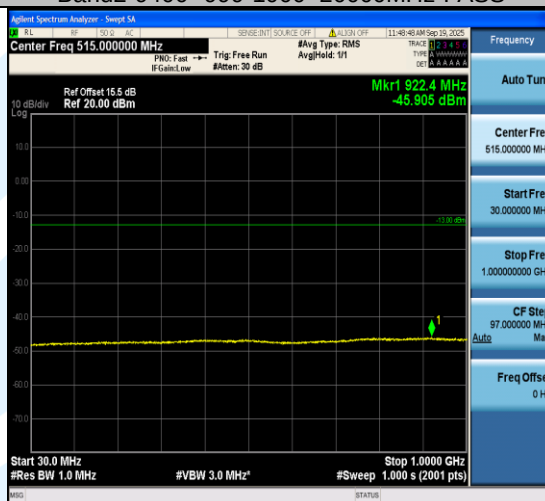
Band2-9538--999-30~1000MHz-PASS
