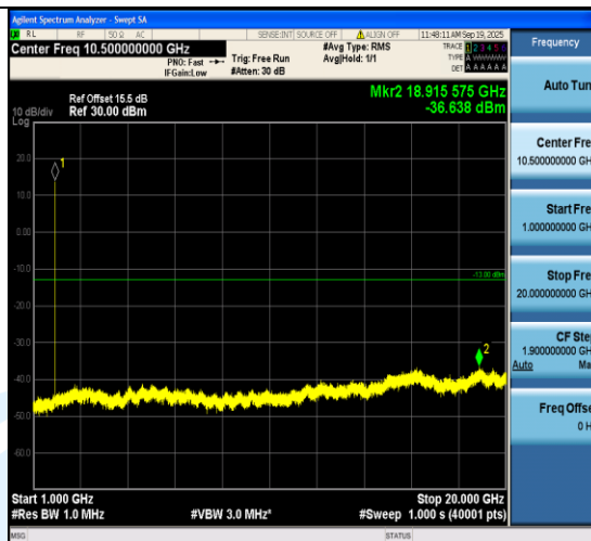
Band2-9400--999-1000~20000MHz-PASS
