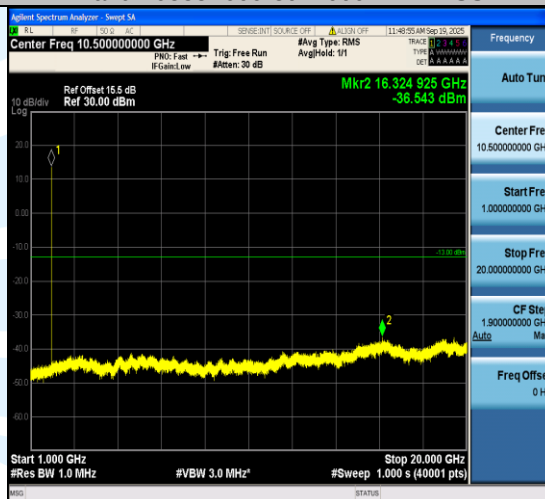
Band2-9538--999-1000~20000MHz-PASS
