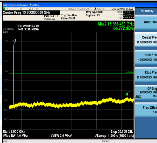
Band4-1513--999-1000~20000MHz-PASS
