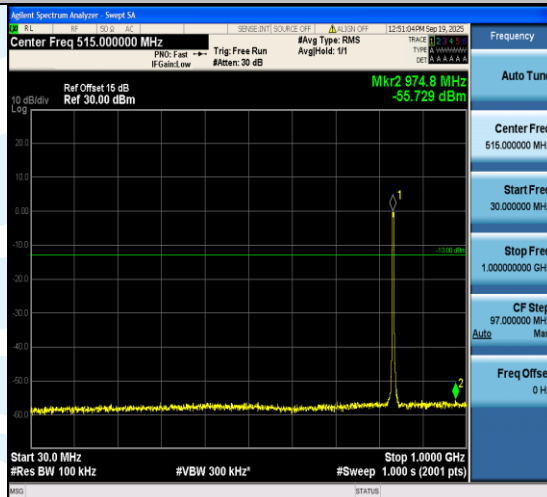
Band5-4182--999-30~1000MHz-PASS
