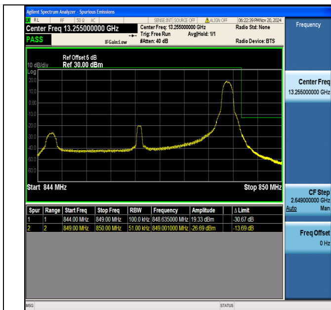
Band5 5MHz QPSK 20625 1RB#24
