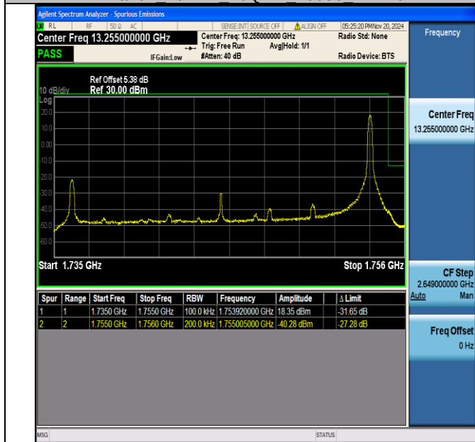
Band4 20MHz 16QAM 20300 1RB#99
