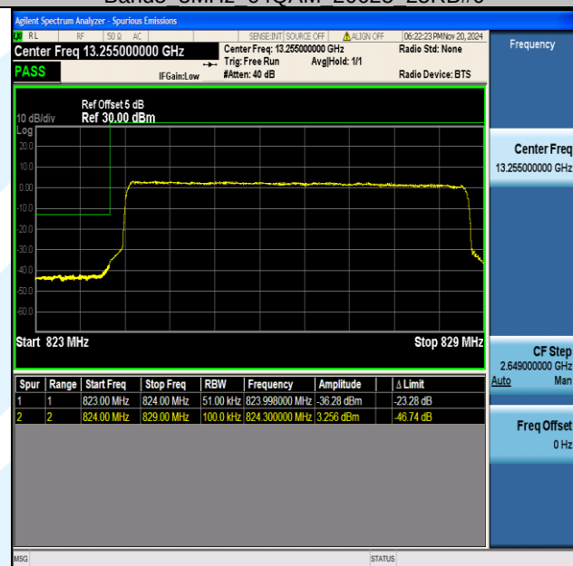
Band5 5MHz 16QAM 20425 25RB#0
