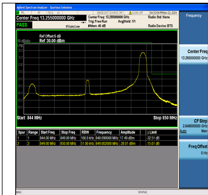
Band5 5MHz 64QAM 20625 1RB#24
