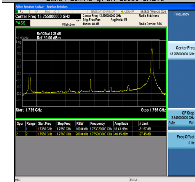
Band4 20MHz QPSK 20300 1RB#99
