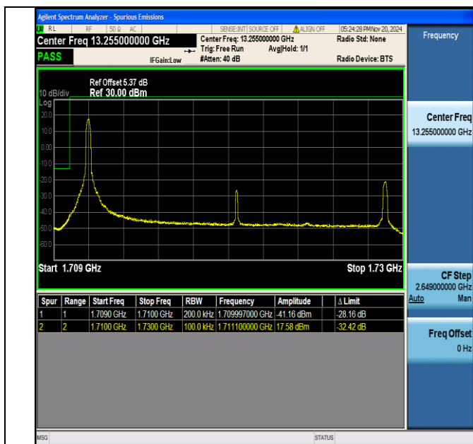
Band4 20MHz 16QAM 20050 1RB#0
