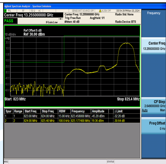
Band5 1.4MHz QPSK 20407 1RB#5
