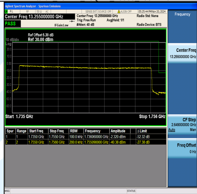
Band4 20MHz 16QAM 20300 100RB#0
