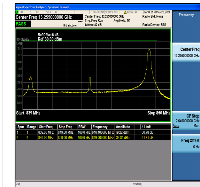
Band5 10MHz QPSK 20600 1RB#49
