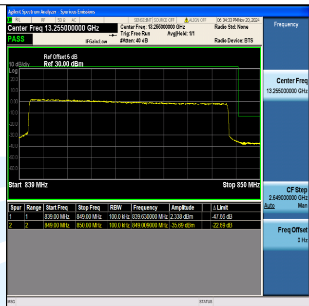
Band5 10MHz QPSK 20600 50RB#0
