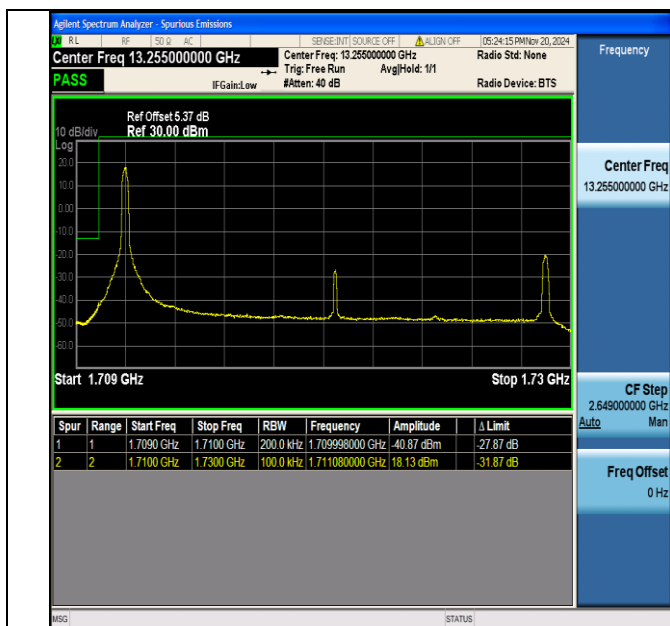
Band4 20MHz QPSK 20050 1RB#0
