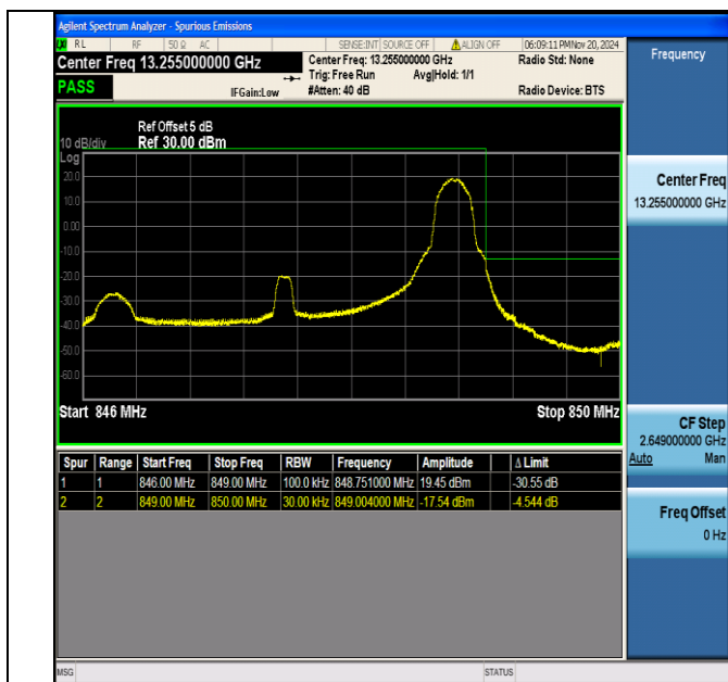
Band5 3MHz QPSK 20635 1RB#14
