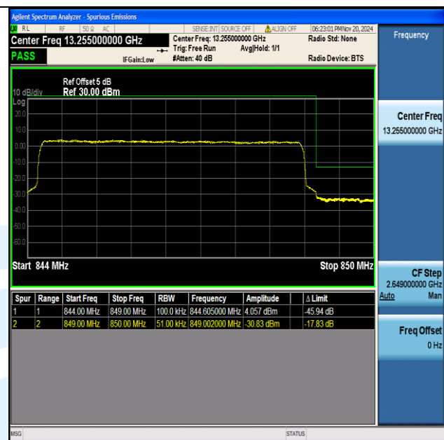
Band5 5MHz QPSK 20625 25RB#0
