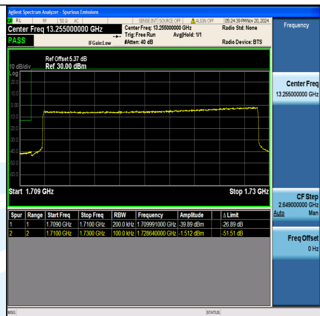
Band4 20MHz QPSK 20050 100RB#0
