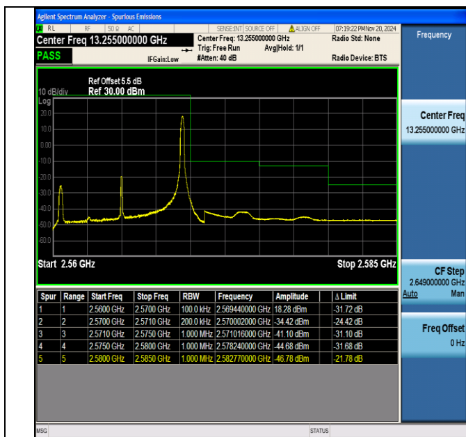
Band7 10MHz QPSK 21400 1RB#49
