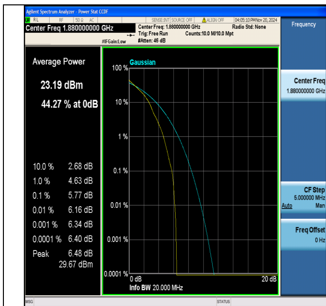
Band2-20MHz-QPSK-18900-1RB#0-PASS
