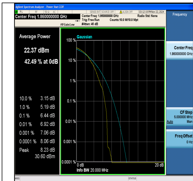
Band2-20MHz-64QAM-18700-1RB#0-PASS
