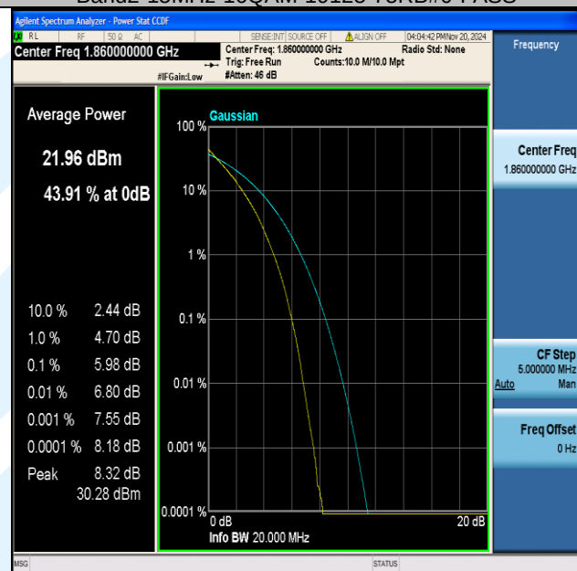
Band2-20MHz-QPSK-18700-100RB#0-PASS
