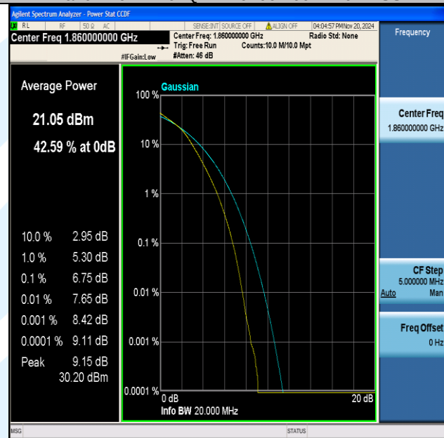
Band2-20MHz-16QAM-18700-100RB#0-PASS
