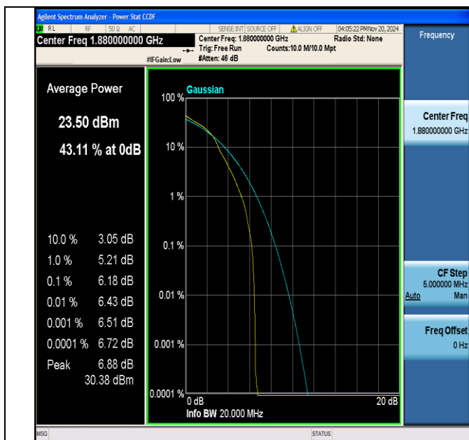
Band2-20MHz-16QAM-18900-1RB#0-PASS
