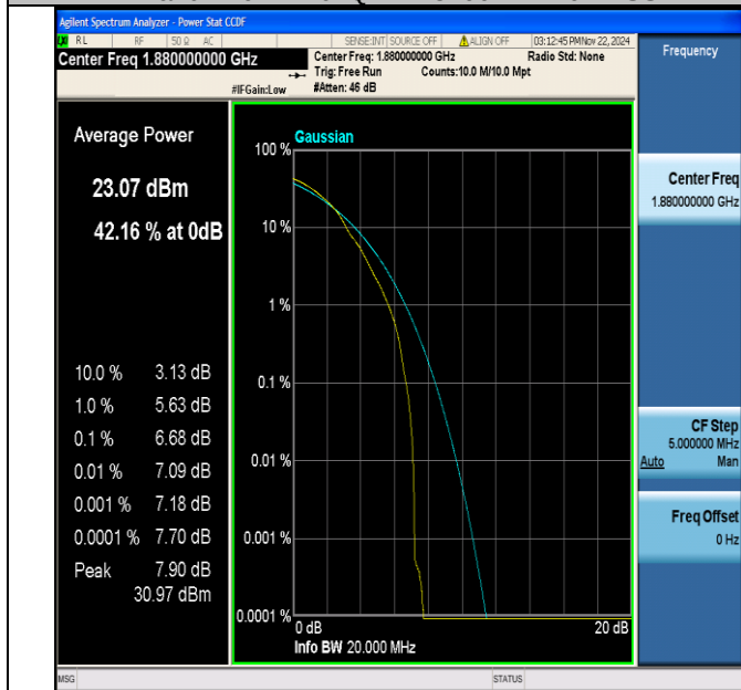
Band2-20MHz-64QAM-18900-1RB#0-PASS
