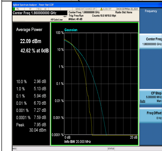
Band2-20MHz-16QAM-18700-1RB#0-PASS
