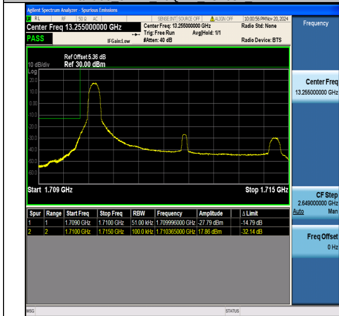
Band66 5MHz QPSK 131997 1RB#0
