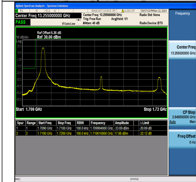
Band66 10MHz 64QAM 132022 1RB#0
