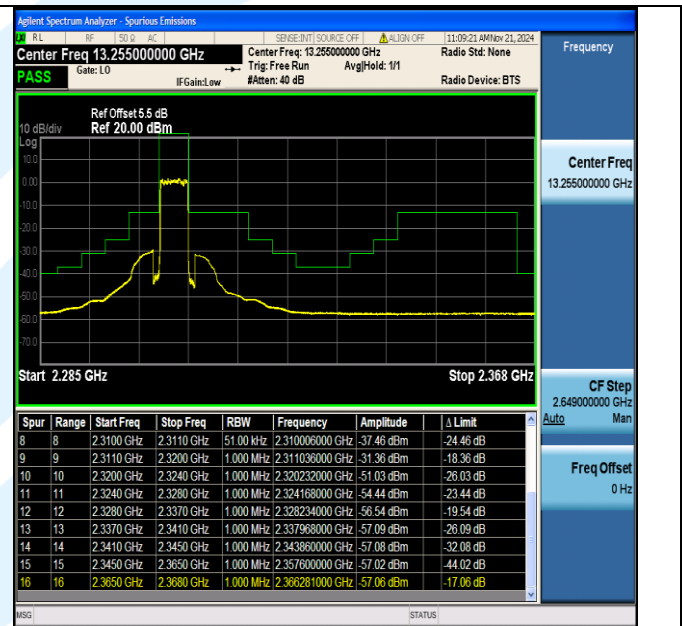
Band40 5MHz QPSK 38725 25RB#0
