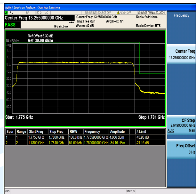
Band66 5MHz QPSK 132647 25RB#0
