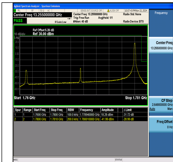
Band66 20MHz 64QAM 132572 1RB#99
