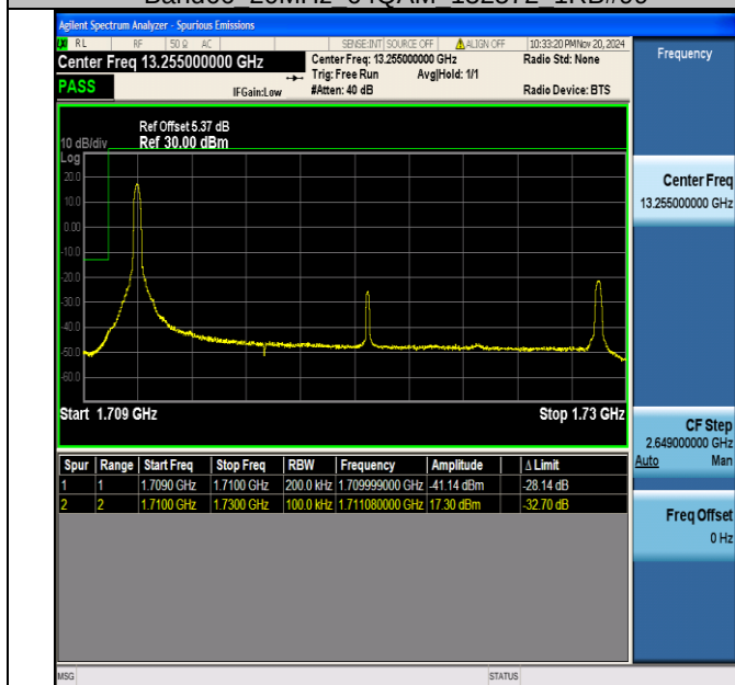
Band66 20MHz 16QAM 132072 1RB#0
