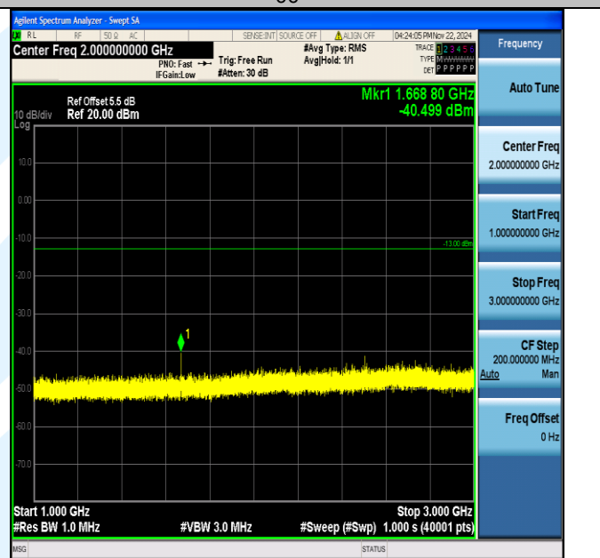
Band5 5MHz 64QAM 20525 1RB#0 1000~3000 1000~3000
