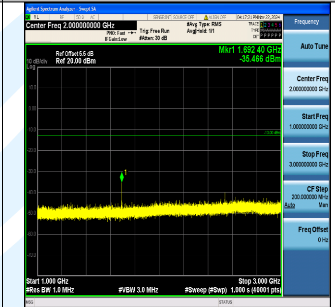
Band5 3MHz 64QAM 20635 1RB#0 1000~3000 1000~3000
