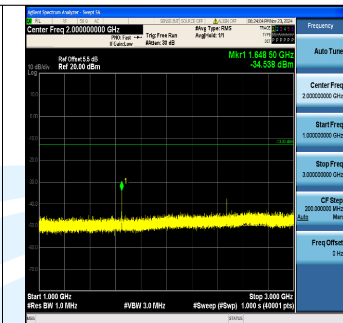
Band5 5MHz 16QAM 20425 1RB#0 1000~3000 1000~3000
