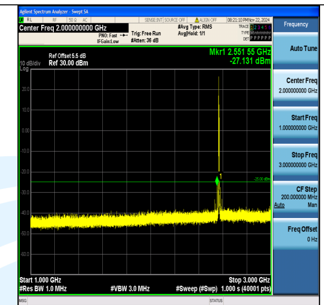
Band7 5MHz 64QAM 21425 1RB#0 1000~3000 1000~3000
