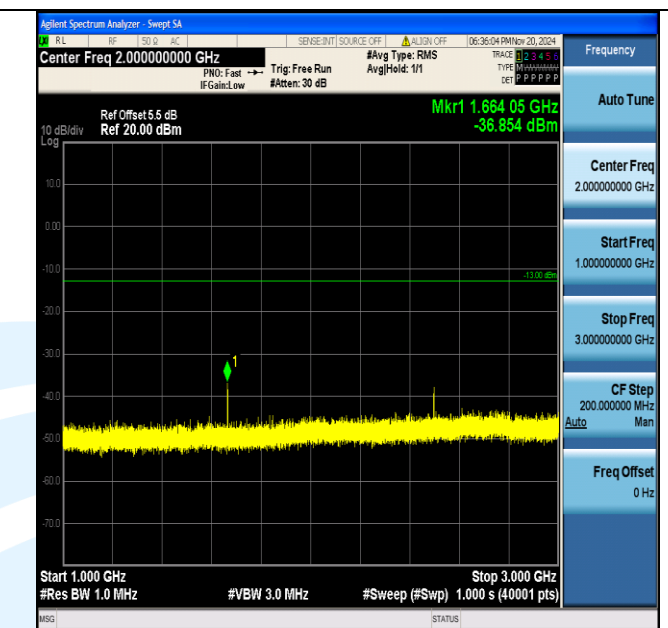
Band5 10MHz QPSK 20525 1RB#0 1000~3000 1000~3000
