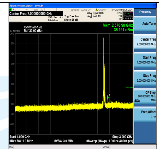
Band7_20MHz_QPSK_20850_1RB#0_1000~3000_1000~3000
