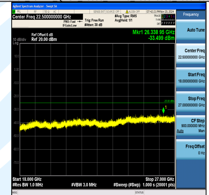
Band7_20MHz_QPSK_20850_1RB#0_18000~27000_18000~27000
