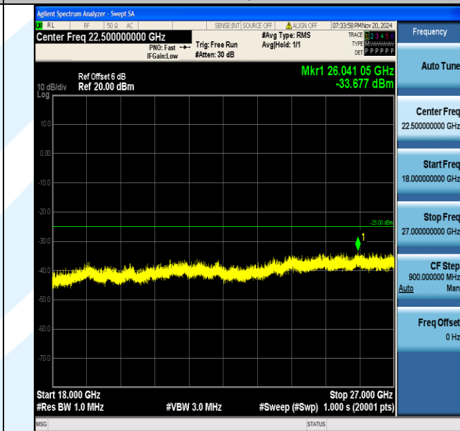
Band7_15MHz_16QAM_21100_1RB#0_18000~27000_18000~27000
