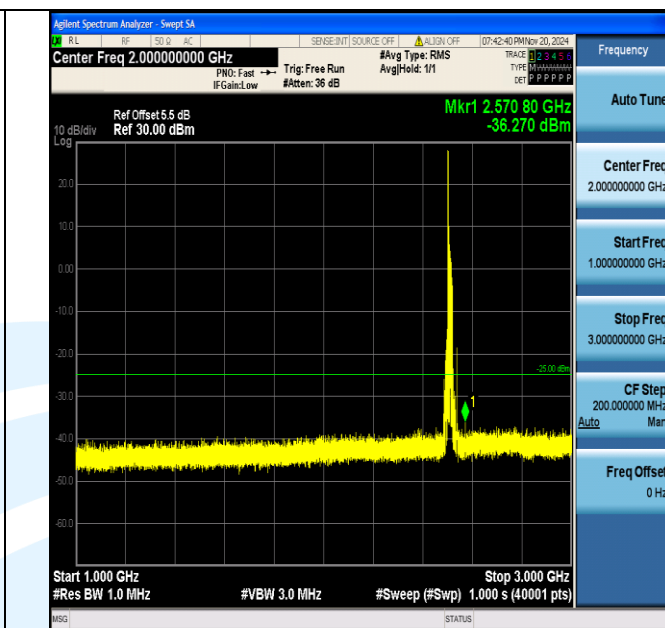
Band7_20MHz_16QAM_20850_1RB#0_1000~3000_1000~3000
