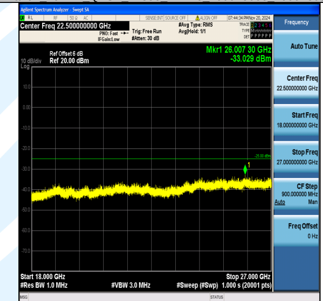
Band7_20MHz_QPSK_21350_1RB#0_18000~27000_18000~27000
