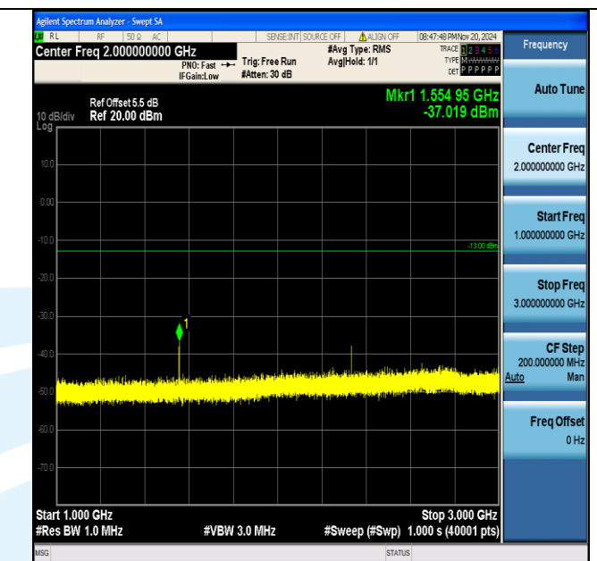
Band13 5MHz QPSK 23205 1RB#0 1000~3000 1000~3000
