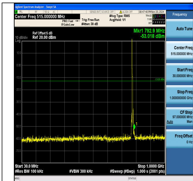
Band13 5MHz QPSK 23205 1RB#0 30~1000 30~1000
