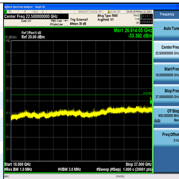
Band38_10MHz_64QAM_38000_1RB#0_18000~27000_18000~27000
