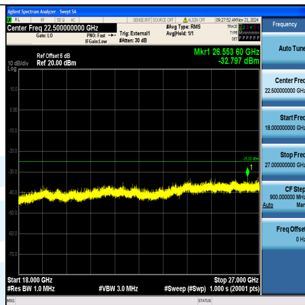
Band38_10MHz_16QAM_38200_1RB#0_18000~27000_18000~27000
