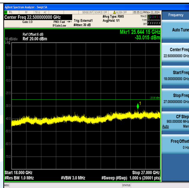
Band38_5MHz_64QAM_38000_1RB#0_18000~27000_18000~27000
