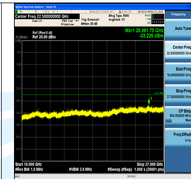
Band38_5MHz_16QAM_38225_1RB#0_18000~27000_18000~27000
