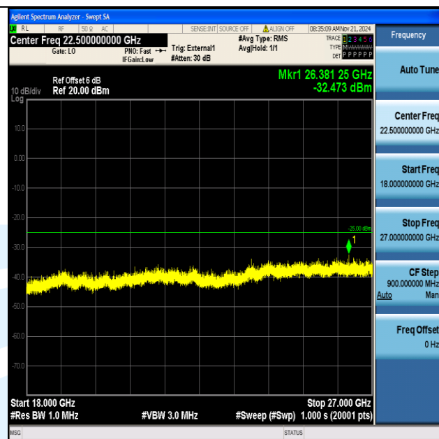
Band38_5MHz_16QAM_38000_1RB#0_18000~27000_18000~27000
