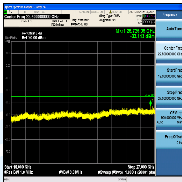
Band38_10MHz_16QAM_38000_1RB#0_18000~27000_18000~27000
