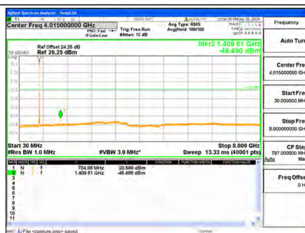
B17 / 10MHz / Low CH / QPSK
