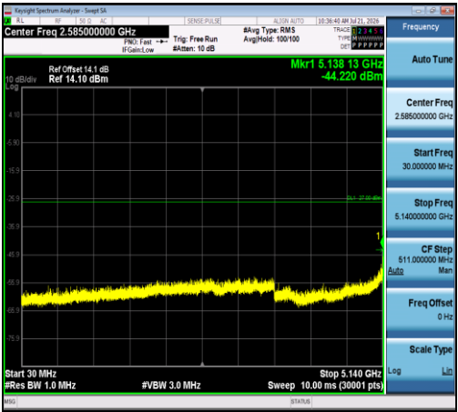
11N40SISO-Ant1-5270-30~5140-PASS
