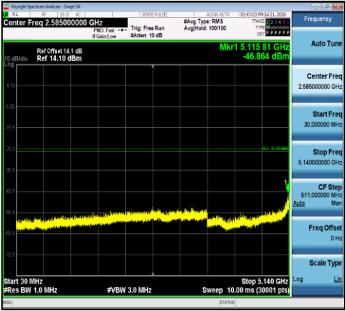
11AC80SISO-Ant1-5290-30~5140-PASS
