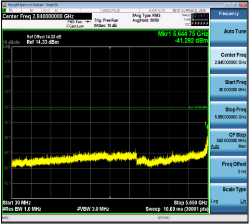
11AC80SISO-Ant1-5775-30~5650-PASS
