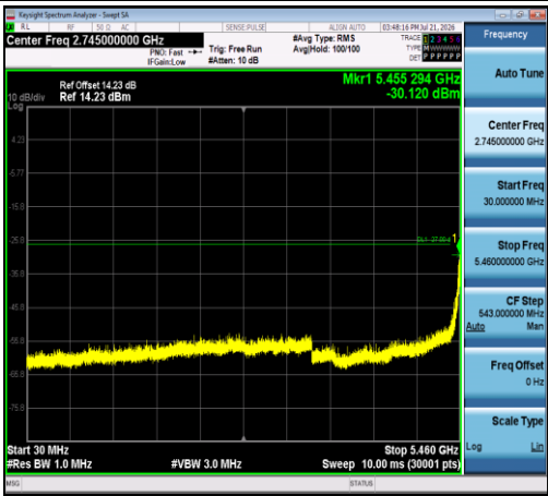
11AC80SISO-Ant1-5530-30~5460-PASS
