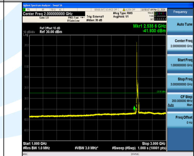
Band38-20MHz-QPSK-37850-1RB#0-1000~3000-PASS
