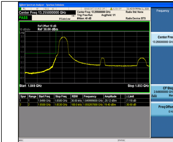
Band2-3MHz-QPSK-18615-1RB#0-PASS
