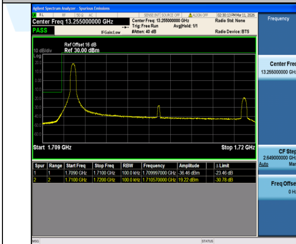
Band4-10MHz-QPSK-20000-1RB#0-PASS
