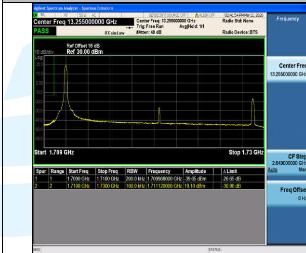
Band4-20MHz-QPSK-20050-1RB#0-PASS
