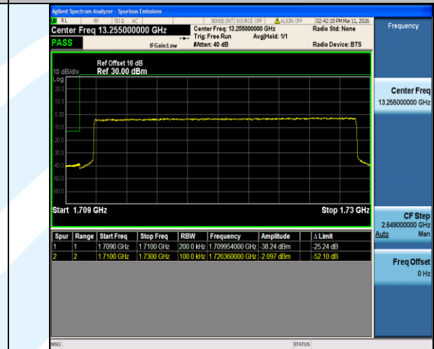
Band4-20MHz-QPSK-20050-100RB#0-PASS
