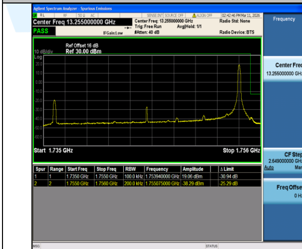
Band4-20MHz-QPSK-20300-1RB#99-PASS
