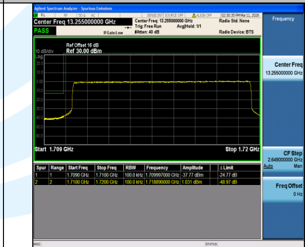
Band4-10MHz-QPSK-20000-50RB#0-PASS
