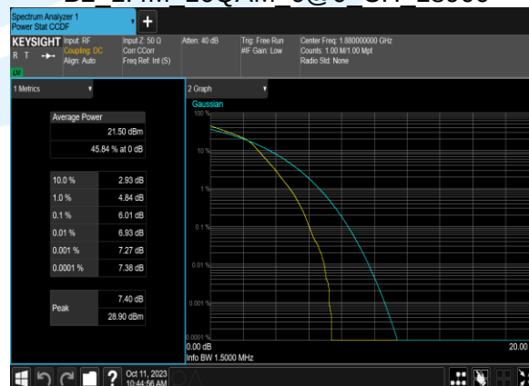
B2_1.4M 16QAM 6@0 CH 18900
