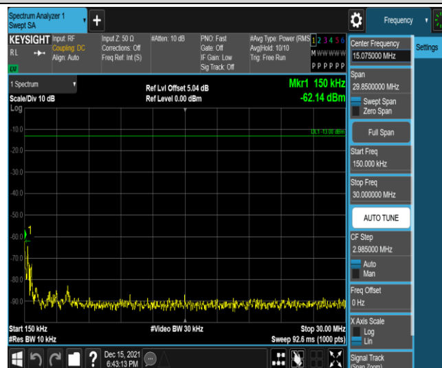
Band12-1.4MHz-QPSK-23095-1RB#0-Range2:0.15~30MHz
