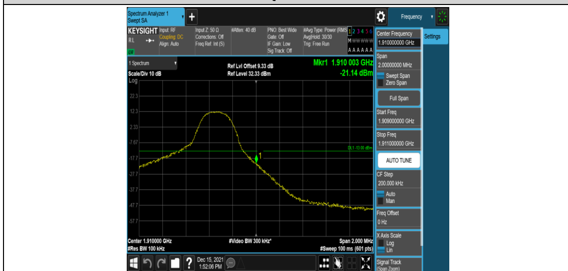
Band2-5MHz-QPSK-19175-1RB#24
