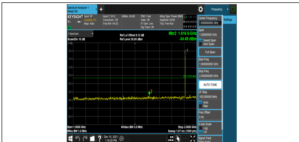
Band2-1.4MHz-QPSK-19193-1RB#0-Range4:1000~2000MHz
