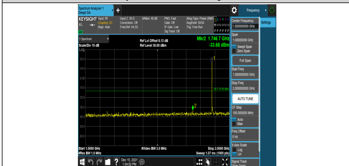
Band2-3MHz-QPSK-18900-1RB#0-Range4:1000~2000MHz
