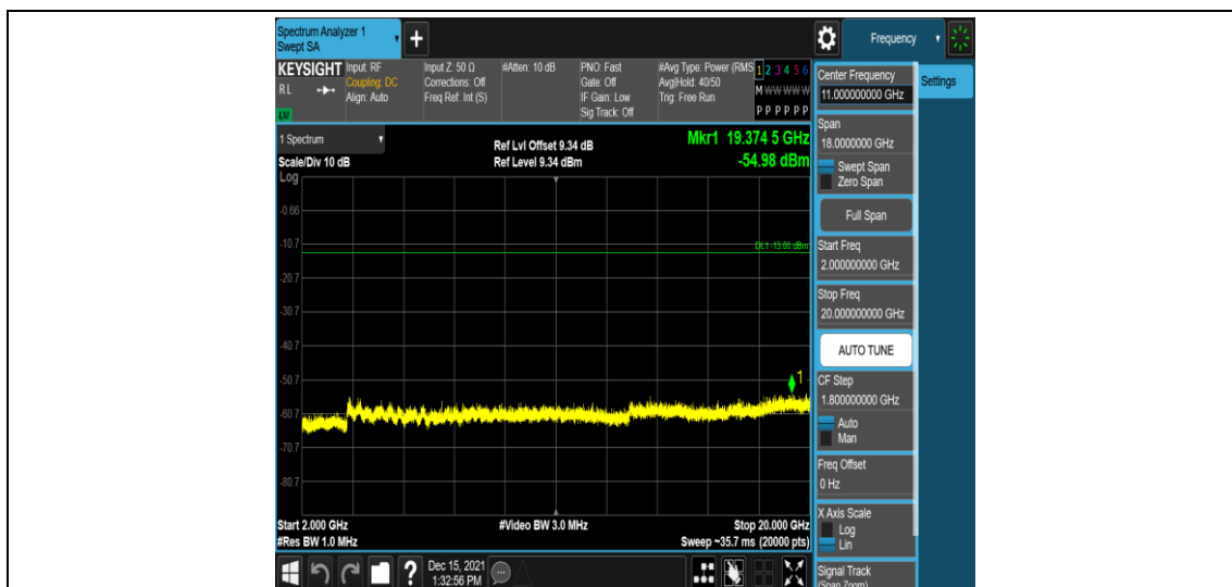
Band2-3MHz-QPSK-18615-1RB#0-Range5:2000~20000MHz
