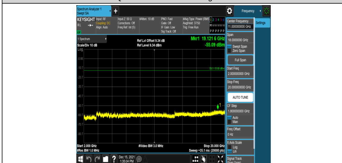
Band2-3MHz-QPSK-18900-1RB#0-Range5:2000~20000MHz
