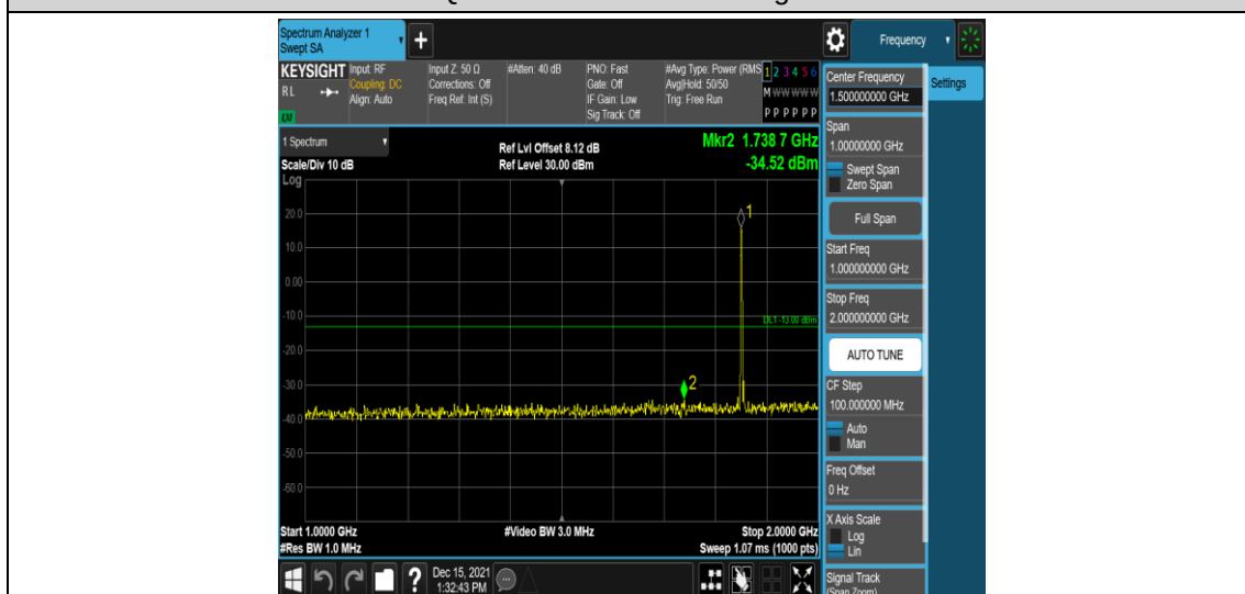
Band2-3MHz-QPSK-18615-1RB#0-Range4:1000~2000MHz
