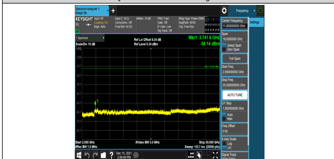
Band2-20MHz-QPSK-18900-1RB#0-Range5:2000~20000MHz
