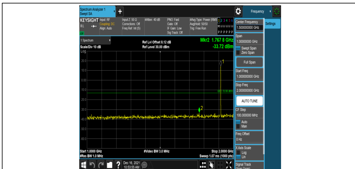
Band25-1.4MHz-QPSK-26683-1RB#0-Range4:1000~2000MHz
