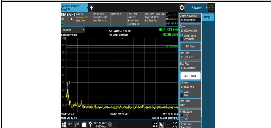
Band25-1.4MHz-QPSK-26683-1RB#0-Range2:0.15~30MHz
