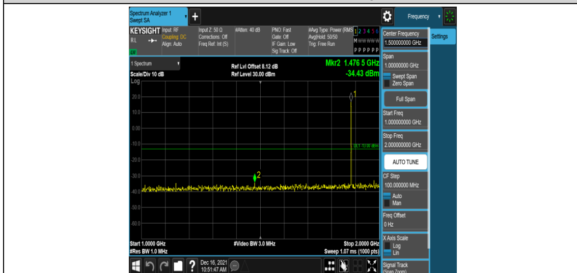
Band25-1.4MHz-QPSK-26365-1RB#0-Range4:1000~2000MHz
