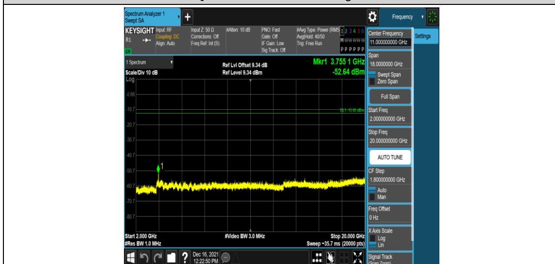
Band25-10MHz-QPSK-26365-1RB#0-Range5:2000~20000MHz
