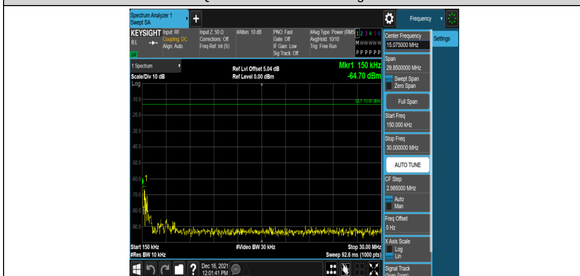
Band25-5MHz-QPSK-26365-1RB#0-Range2:0.15~30MHz
