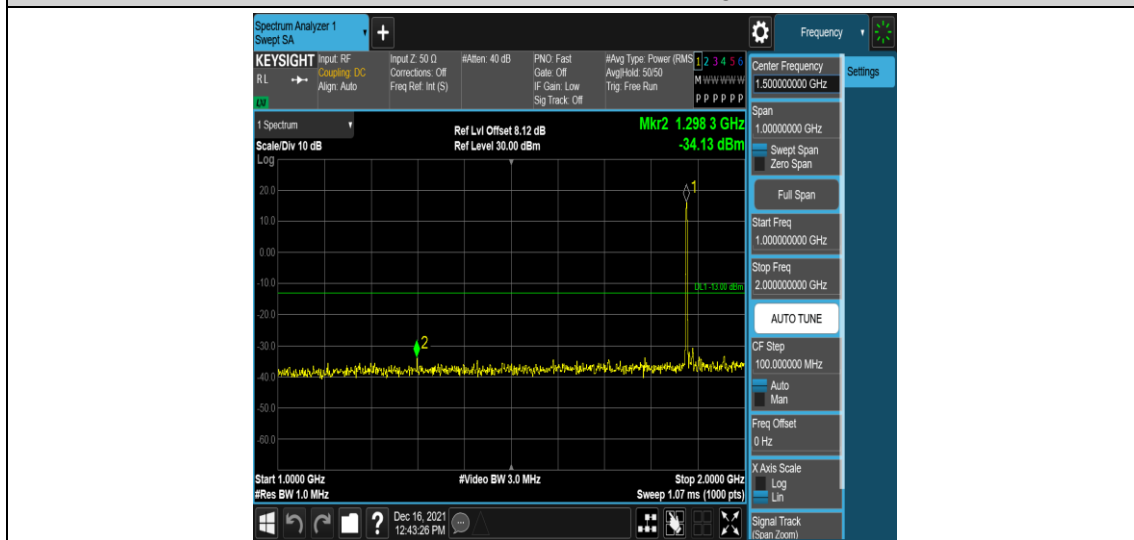
Band25-15MHz-QPSK-26365-1RB#0-Range4:1000~2000MHz
