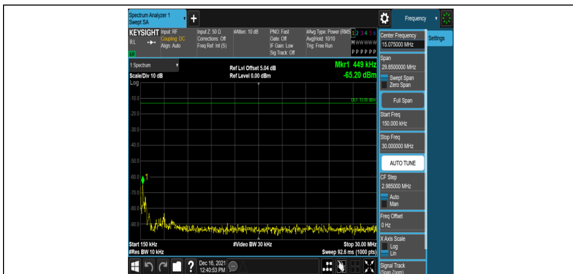
Band25-15MHz-QPSK-26115-1RB#0-Range2:0.15~30MHz
