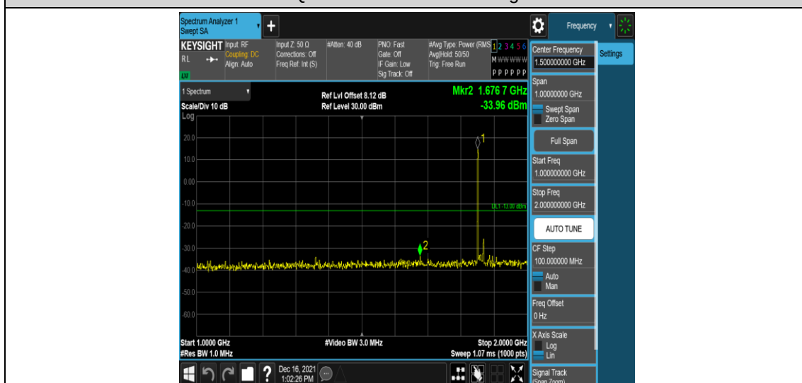
Band25-20MHz-QPSK-26140-1RB#0-Range4:1000~2000MHz
