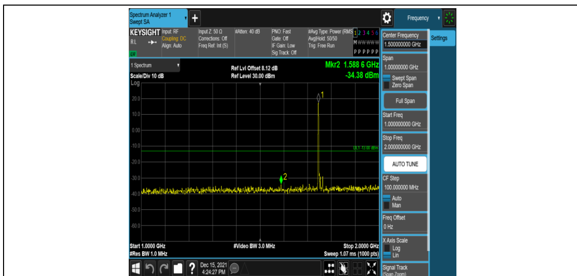
Band4-10MHz-QPSK-20350-1RB#0-Range4:1000~2000MHz
