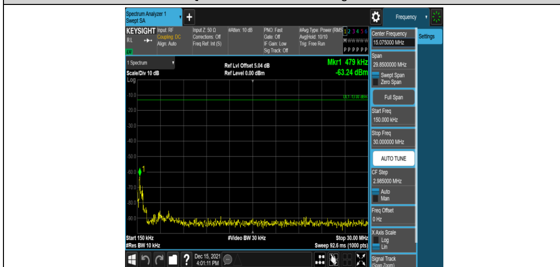
Band4-5MHz-QPSK-20175-1RB#0-Range2:0.15~30MHz
