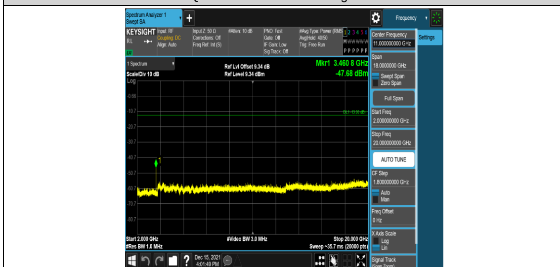
Band4-5MHz-QPSK-20175-1RB#0-Range5:2000~20000MHz
