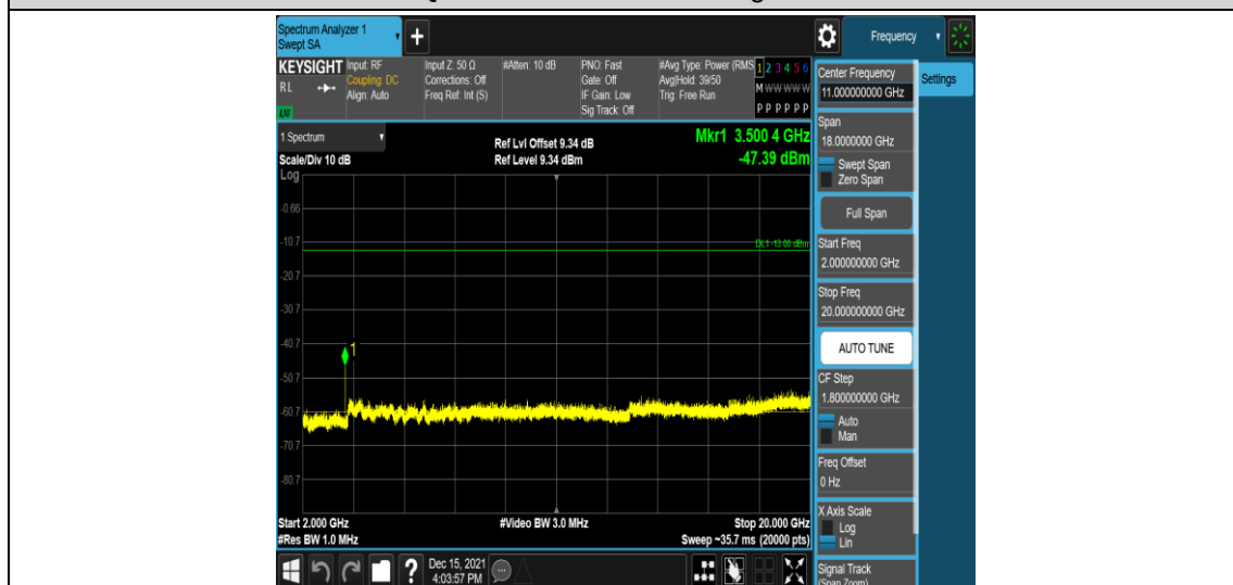
Band4-5MHz-QPSK-20375-1RB#0-Range5:2000~20000MHz
