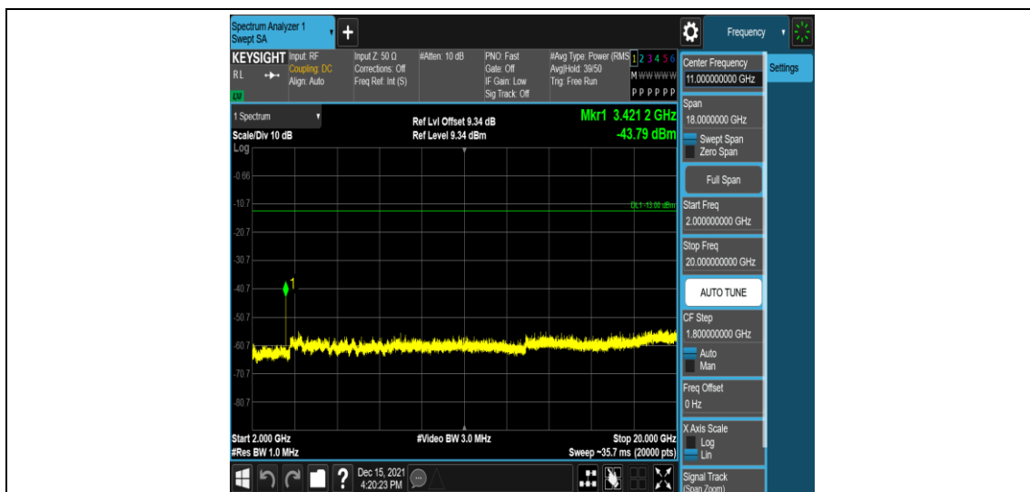
Band4-10MHz-QPSK-20000-1RB#0-Range5:2000~20000MHz
