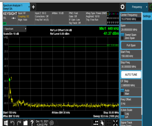
Band4-10MHz-QPSK-20350-1RB#0-Range2:0.15~30MHz
