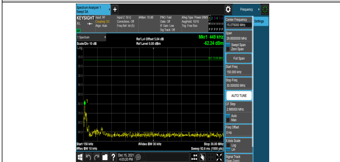
Band4-5MHz-QPSK-20375-1RB#0-Range2:0.15~30MHz
